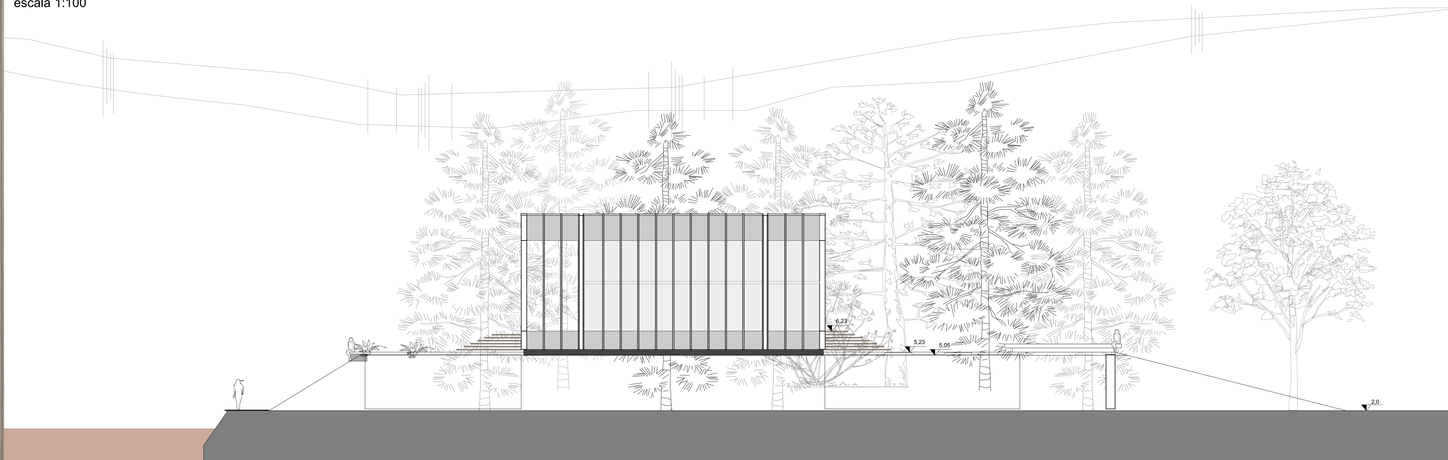
VISTA NOVA ENTRADA escala 1:100
