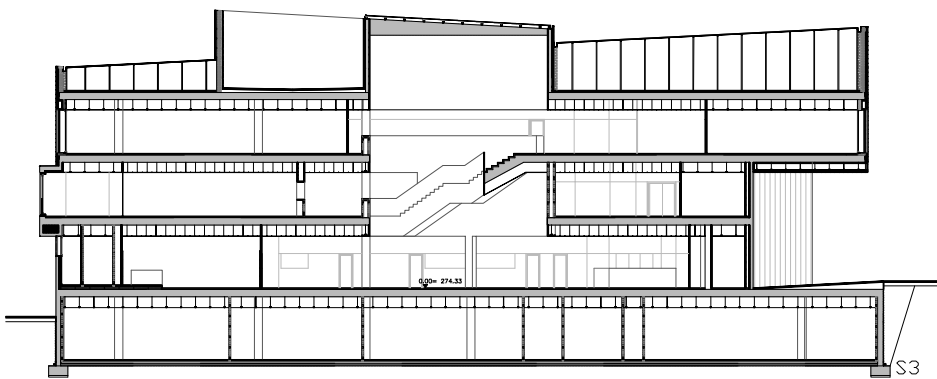
SECCIÓN PATIO INTERIOR
