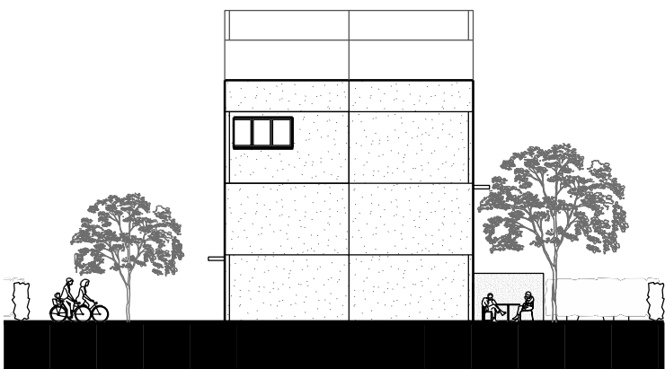
FACADE NORD
