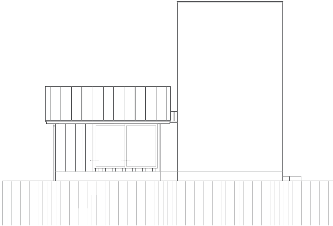
Elevation 1:100
