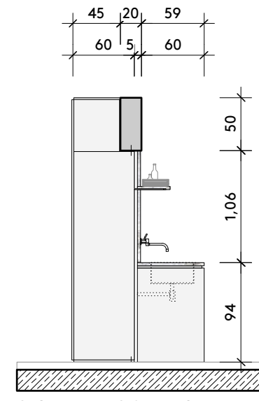
Schnitt EBS & Küche
