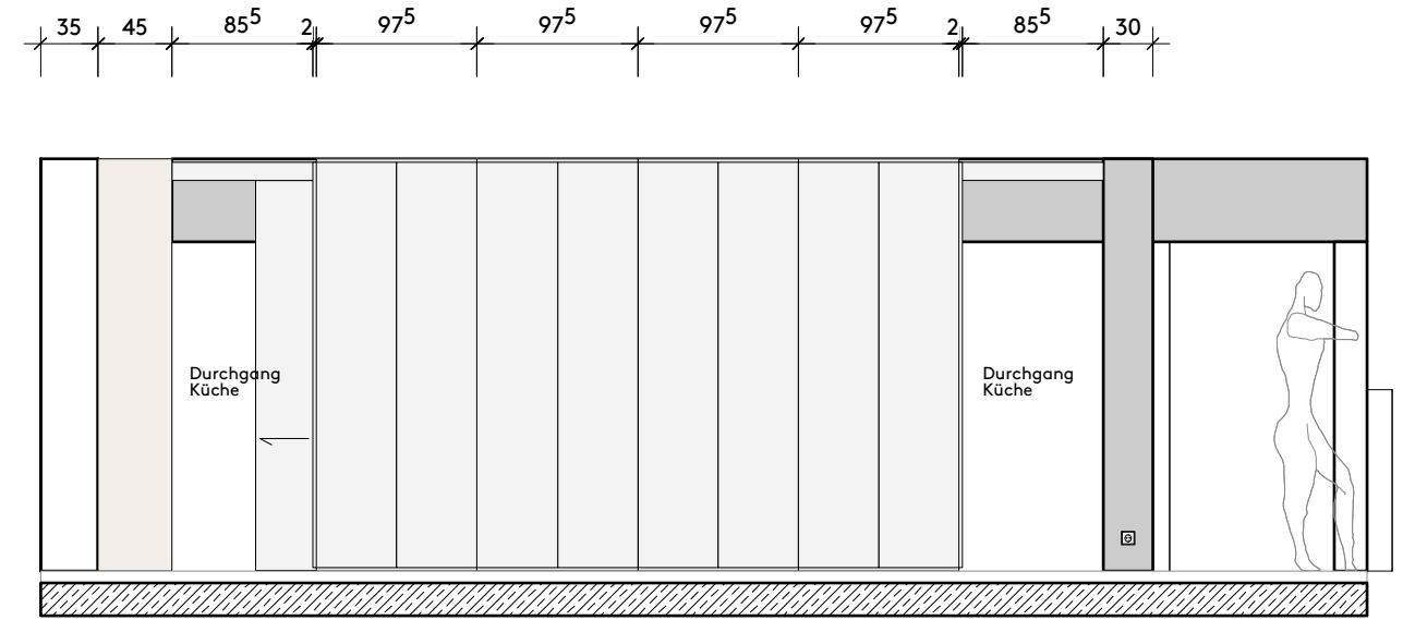
Ansicht Schaf und Badezimmer
