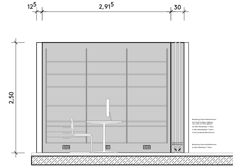
Ansicht Regal Arbeitszimmer
