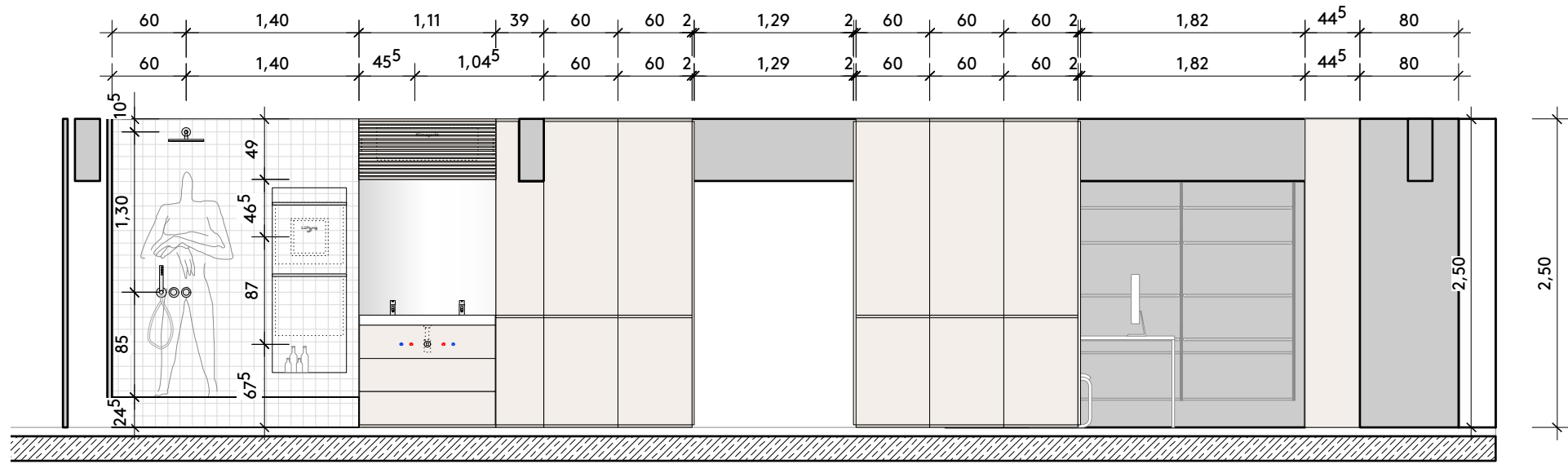
Ansicht Badezimmer & Einbauschränk (Türen offen)
