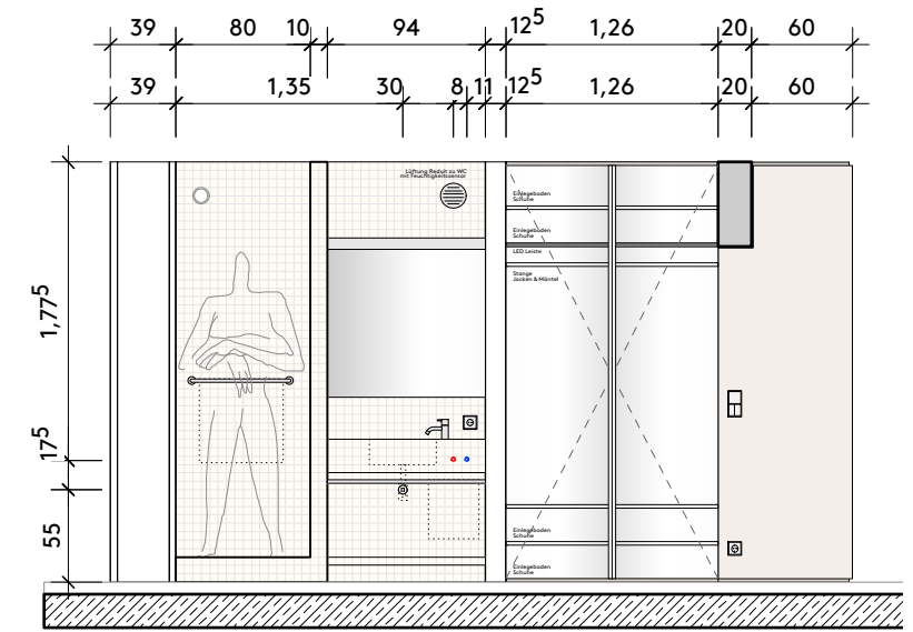
Ansicht Regal Waschtisch
