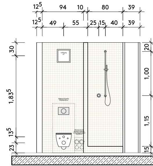
Ansicht WC & Dusche
