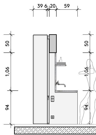
Ansicht EBS & Küche
