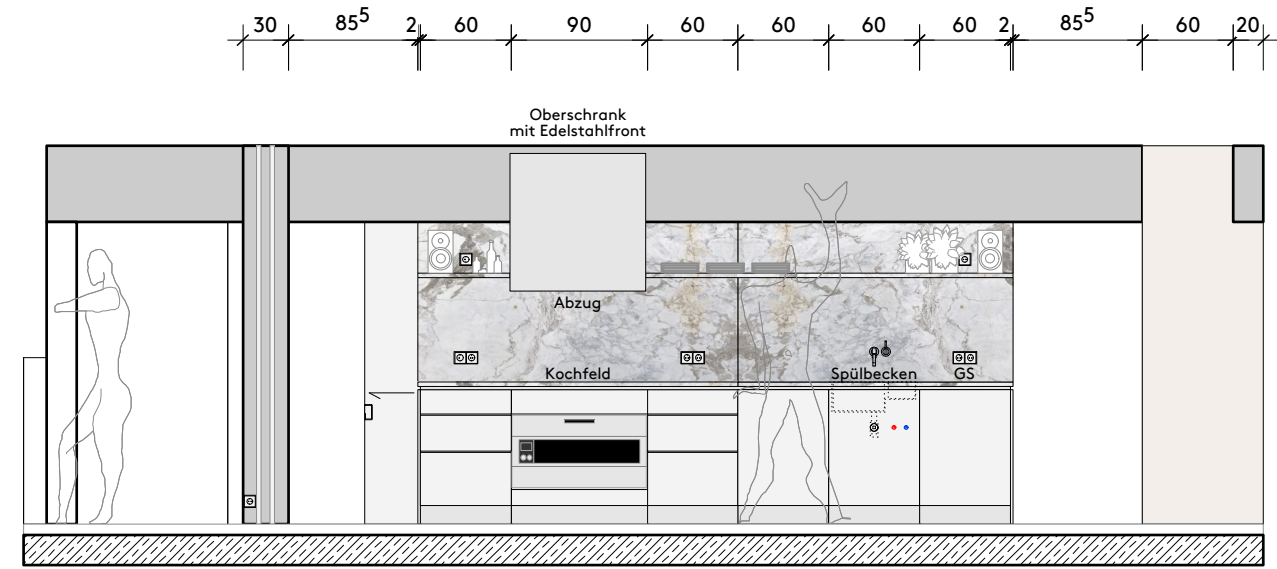
Ansicht Küche mit Durchgang in Schlaf- und Badezimmer
