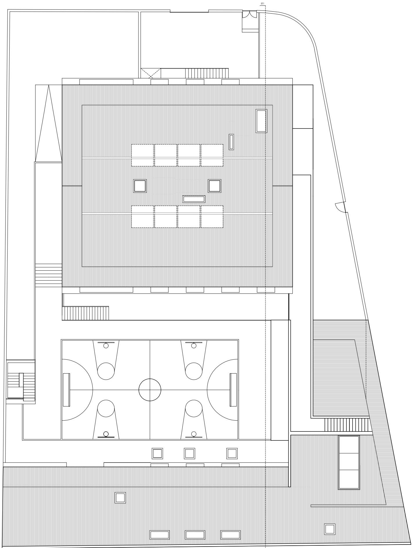
planta de cobertura
