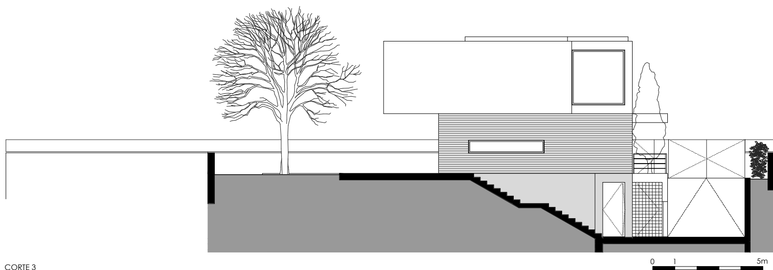
CORTE 3
