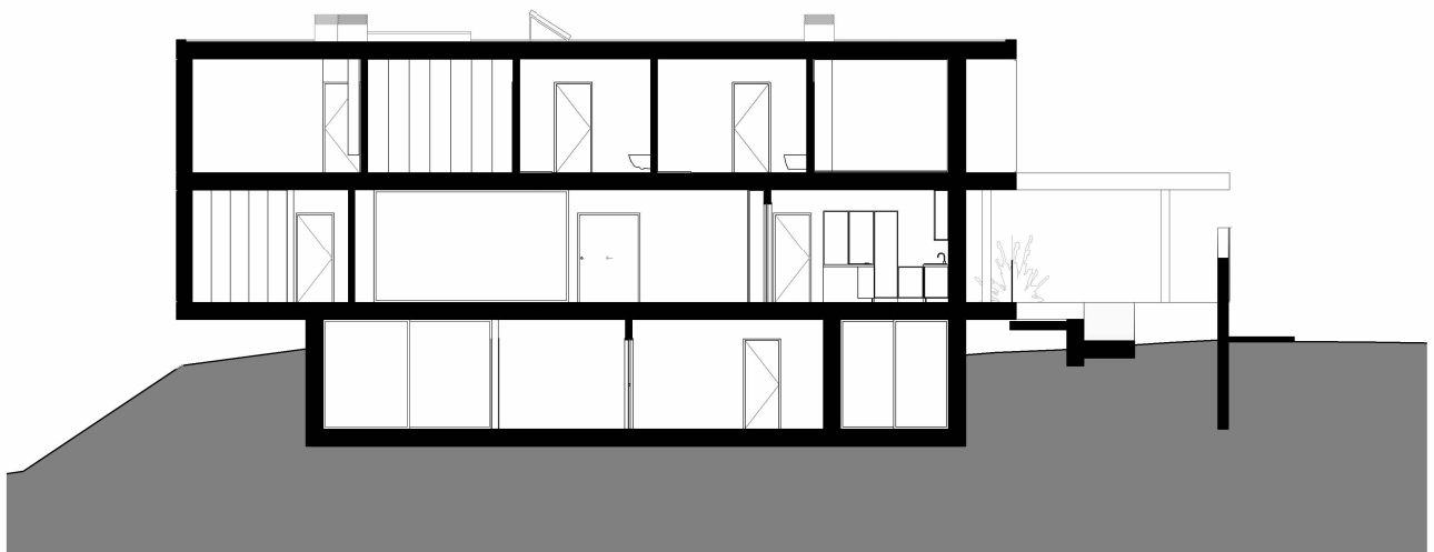
CORTE 2
