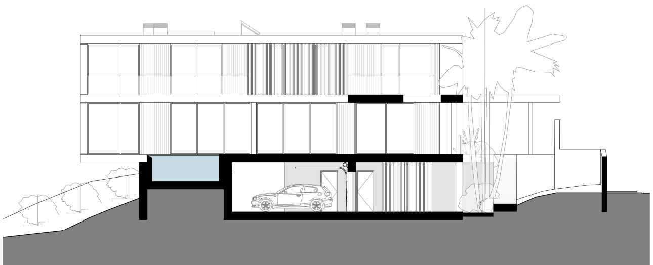
CORTE 3
