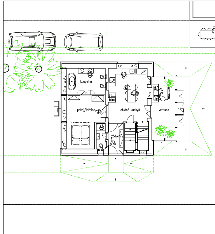
půdorys přízemí
