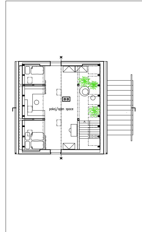
půdorys podkroví
