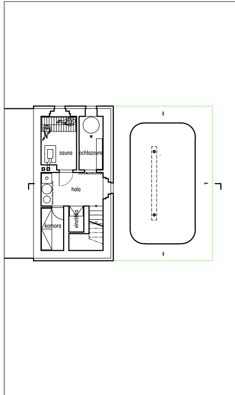
půdorys polosuterénu
