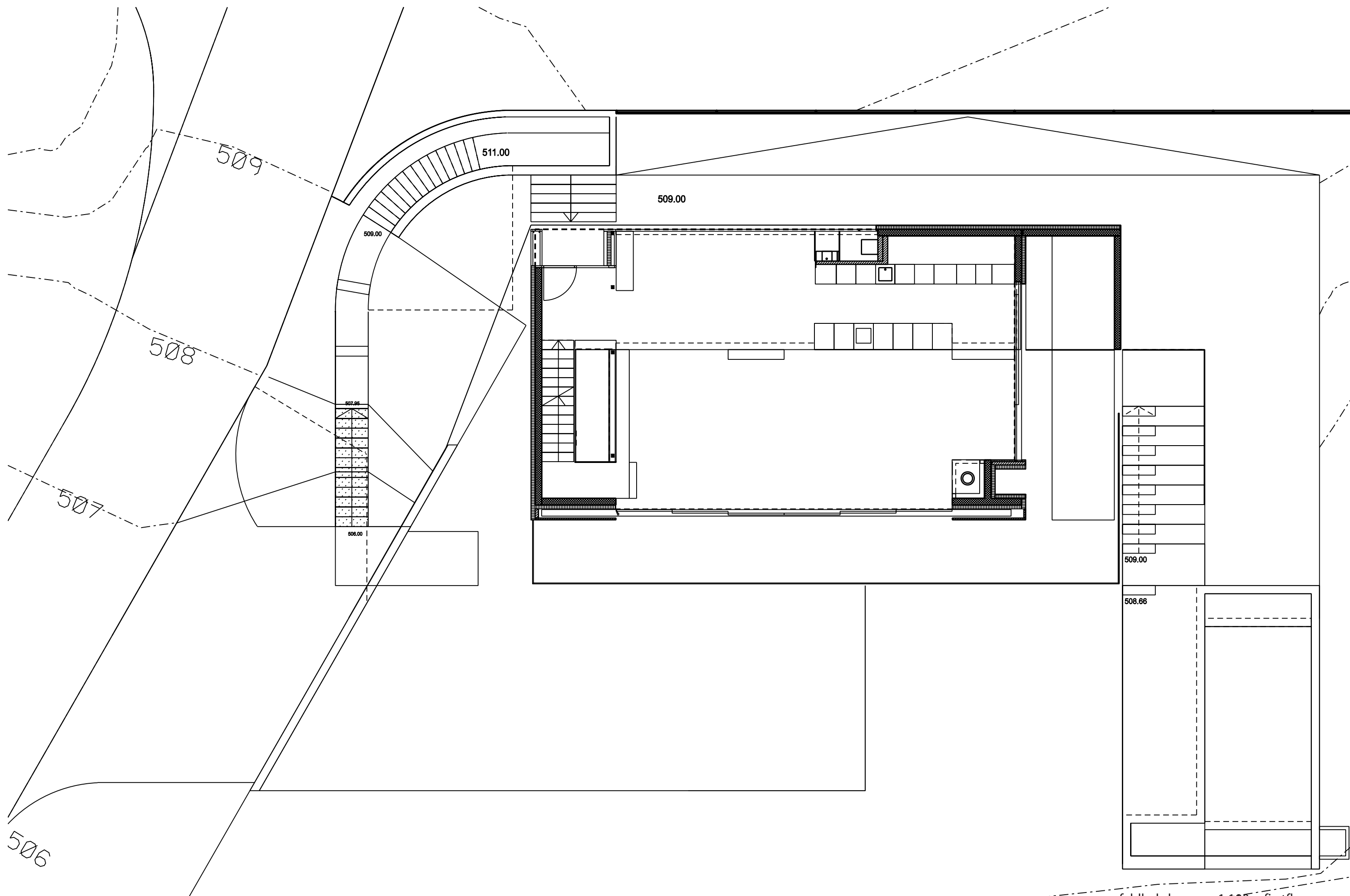
feldbalz house 1:100 firstfloor gus wüstemann ma eth sia coac
