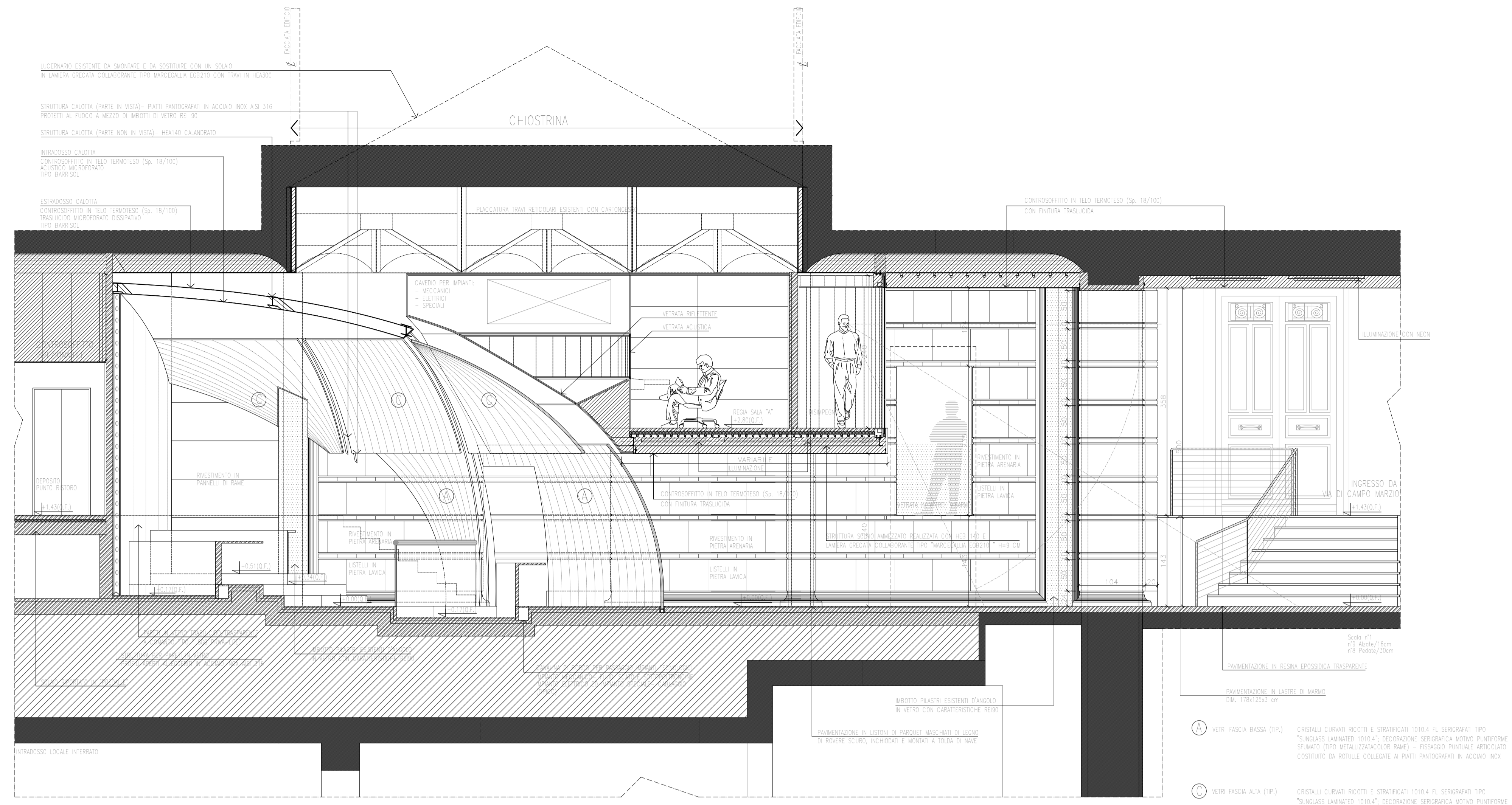
SEZIONE TRASVERSALE B-B Rapp. 1:50
