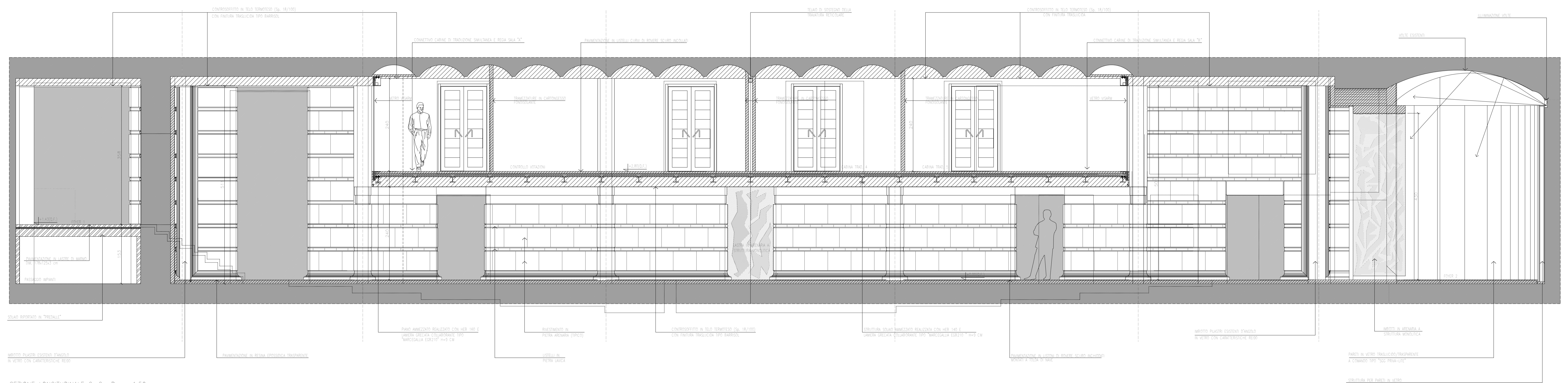
SEZIONE LONGITUDINALE C-C Rapp. 1:50
