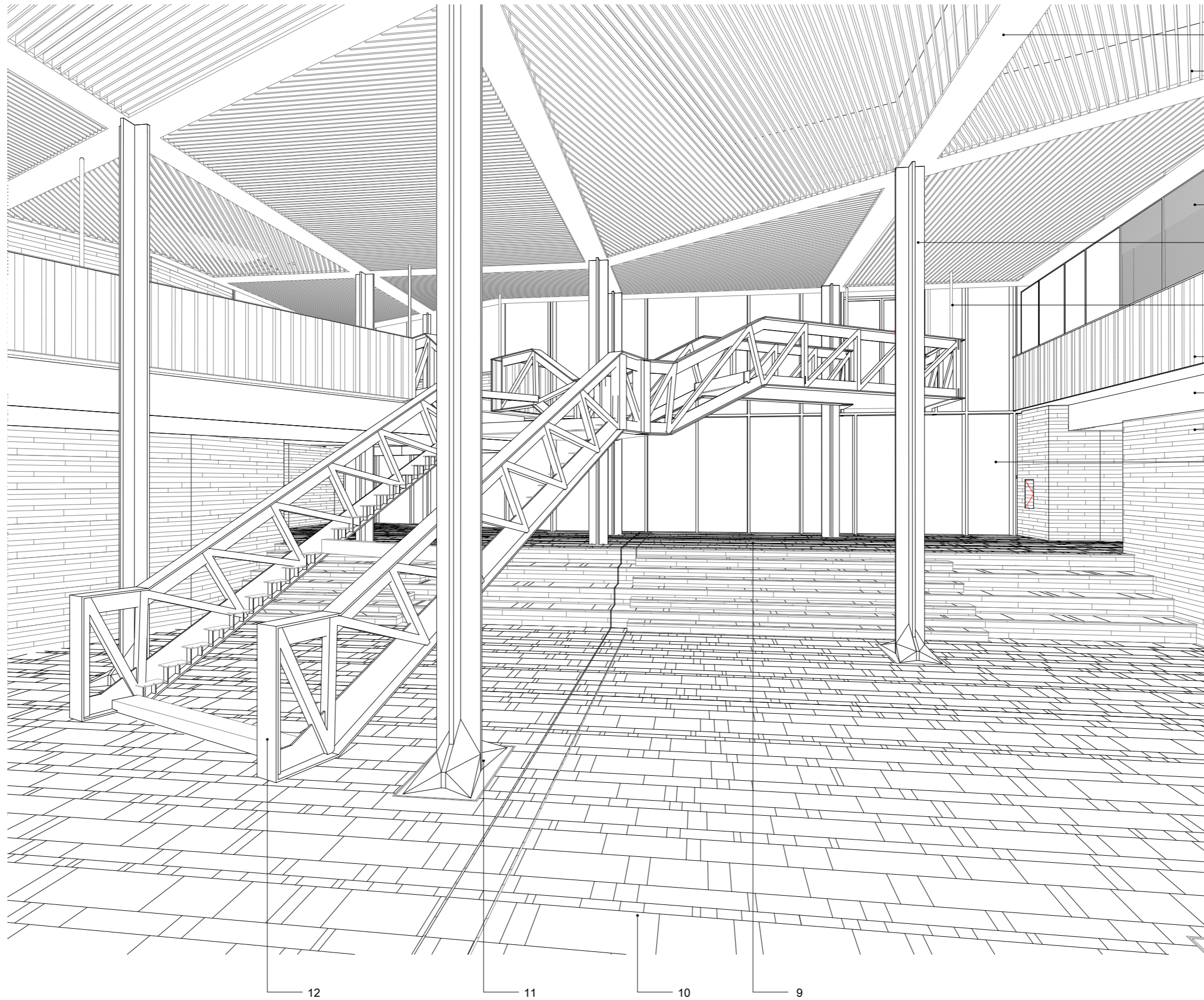
Détail 3 : Détail escalier principal - Vue sans finitions
