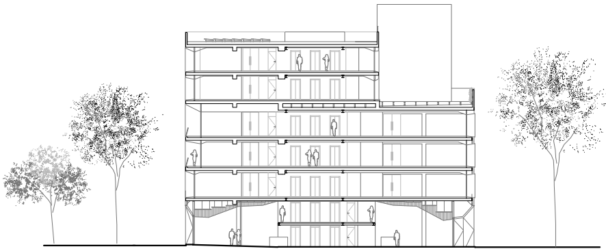
Sección Transversal. Cross Section
