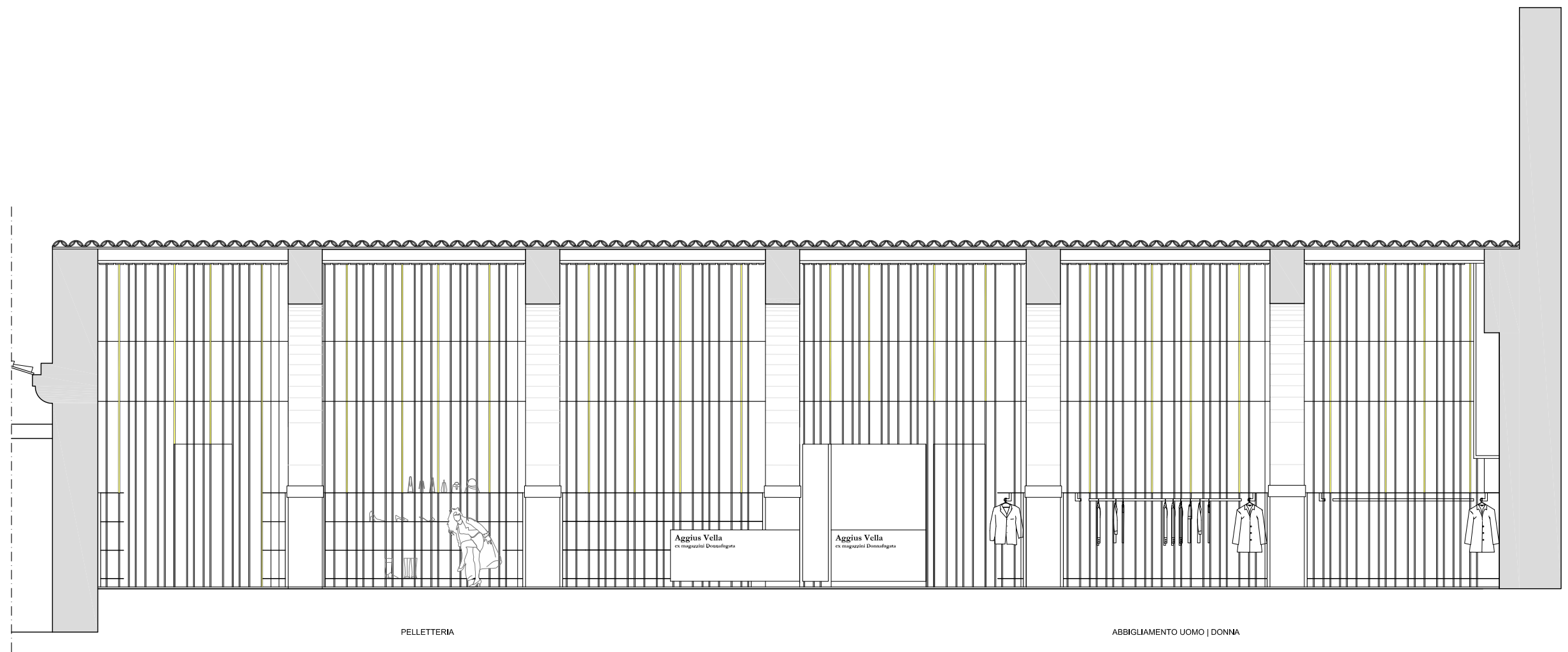
SEZIONE A-A'
