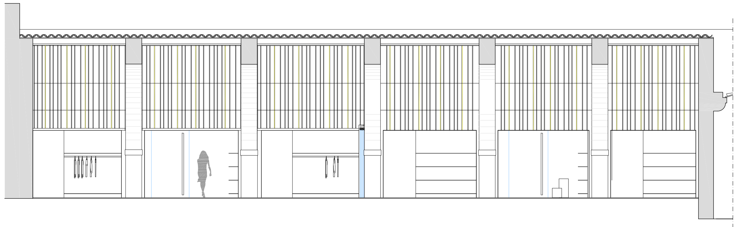
SEZIONE B-B'
