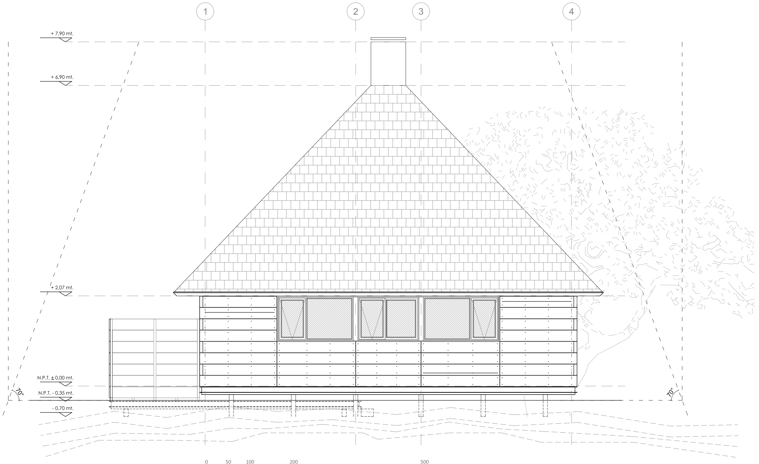
elevación norte
