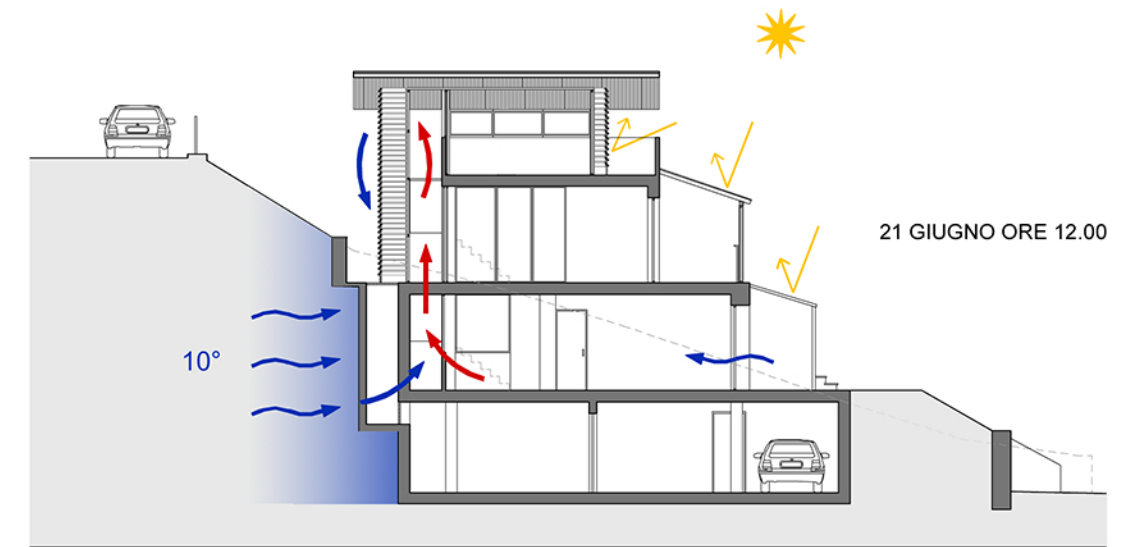
SOLEGGIAMENTO ESTIVO
