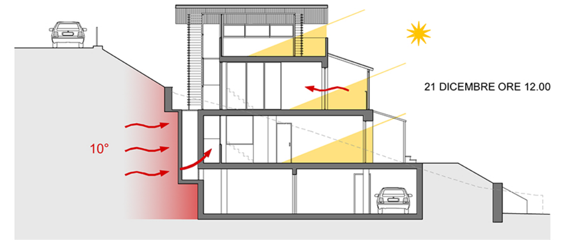
SOLEGGIAMENTO INVERNALE
