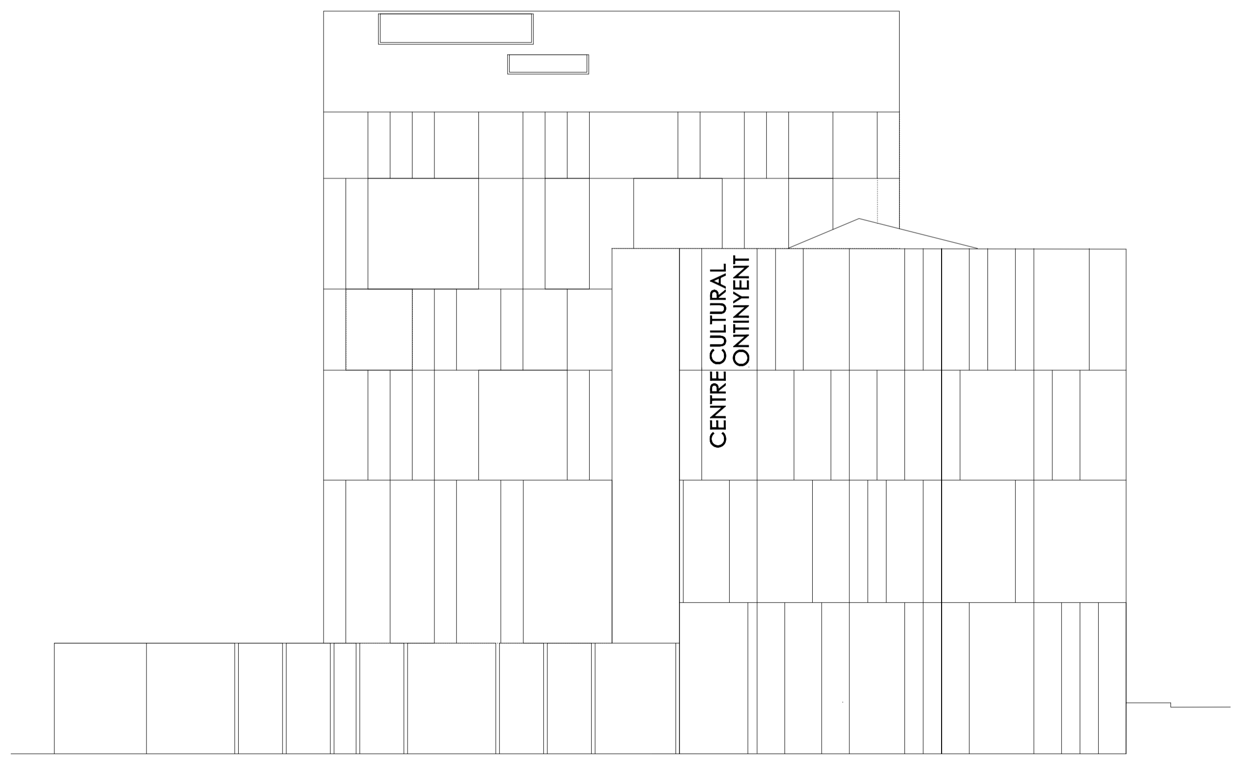
ALZADO NOROESTE 0 5
