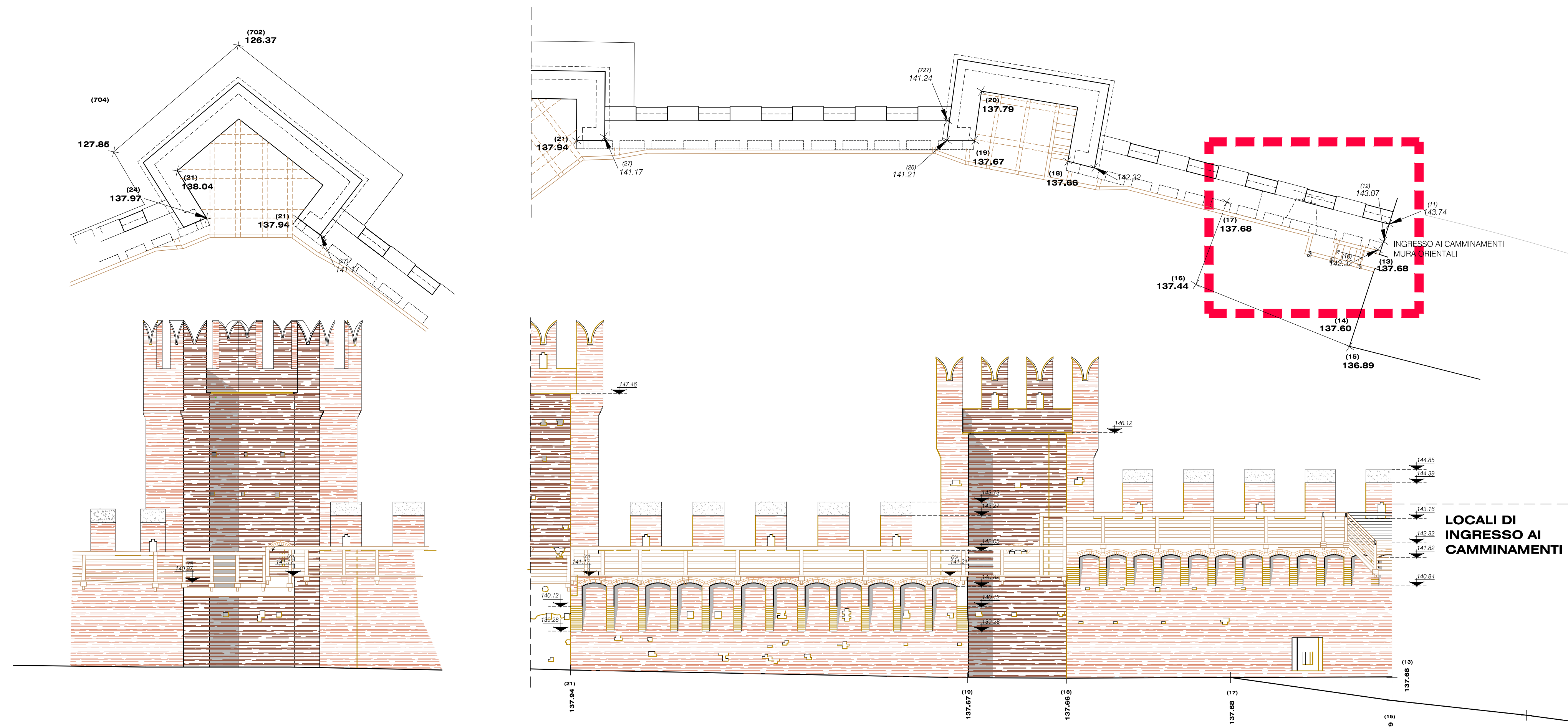
REALIZZAZIONE NUOVI CAMMINAMENTI PROSPETTO INTERNO 1-1
