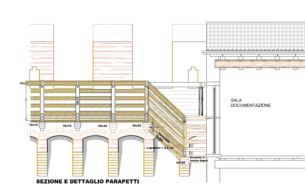
SEZIONE E DETTAGLIO PARAPETTI
