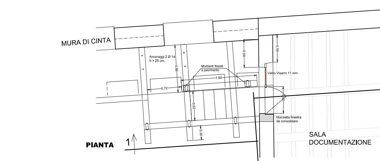
COLLEGAMENTO AI NUOVI PERCORSI DALLA SALA DOCUMENTAZIONE PIANTA PROSPETTO SEZIONE
