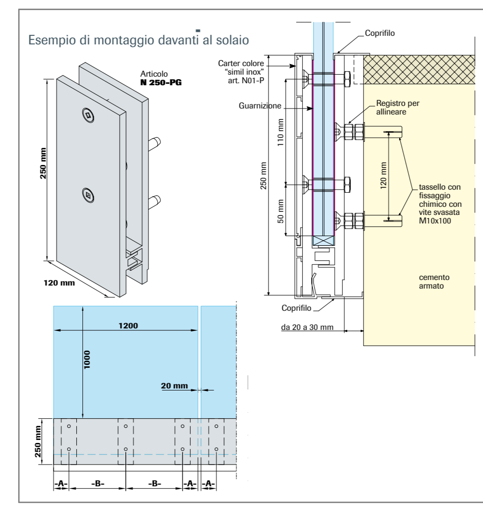
BALAUSTRA IN VETRO TEMPERATO TRASPARENTE CORRIMANO DI ACCIAIO NIKELATO O LEGNO NATURALE d.mmm55
