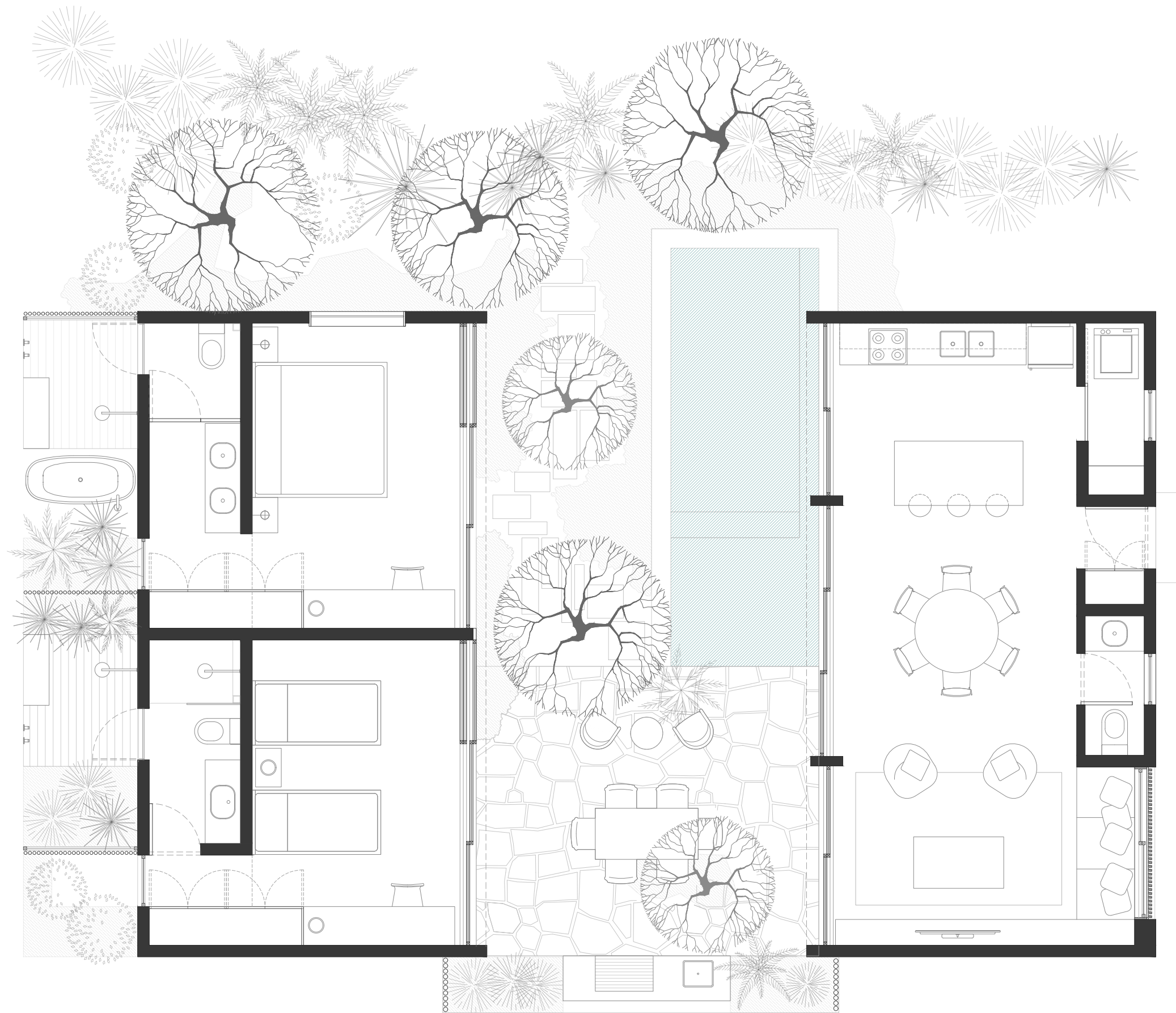
Planta Baja | Villa 04 BRUMA
