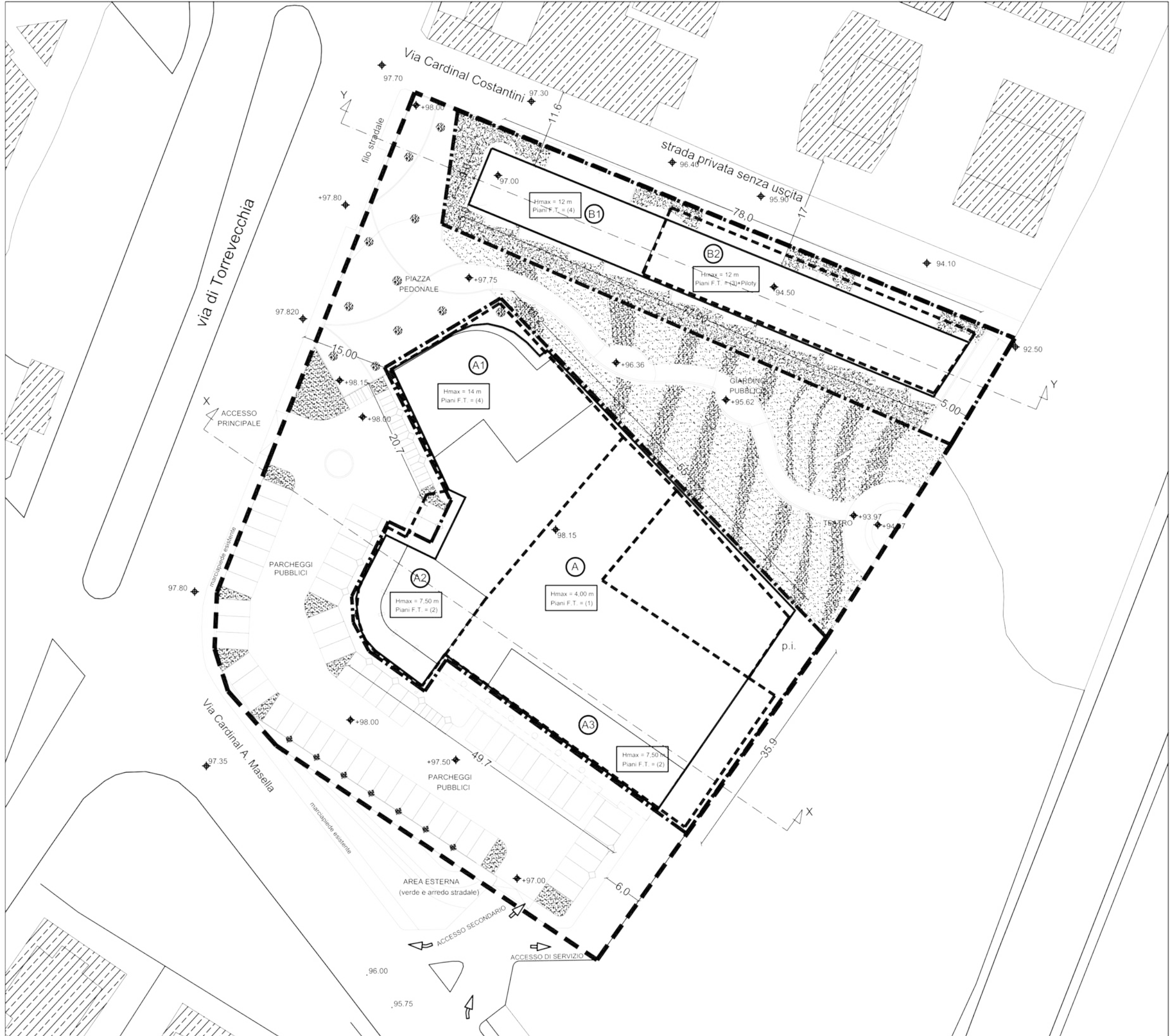
PLANIVOLUMETRICO ESECUTIVO rapp. 1:500
