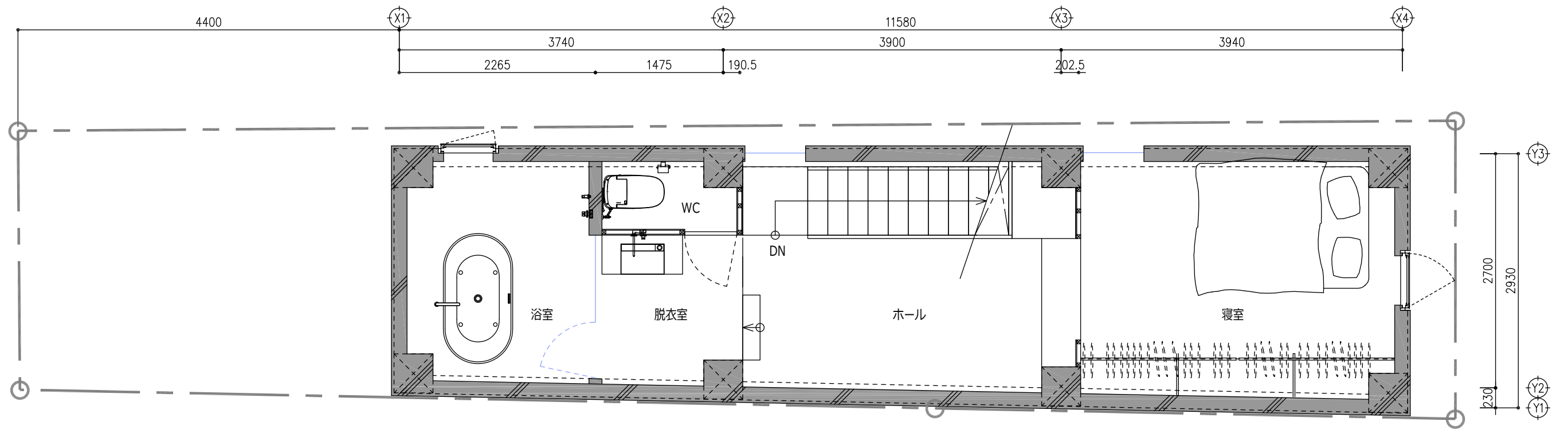
2階平面図
