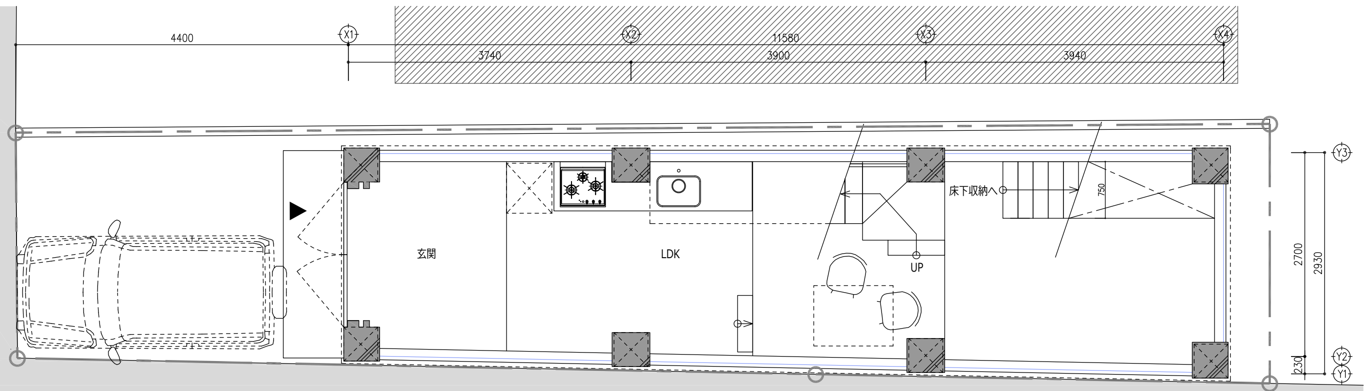
1階平面図
