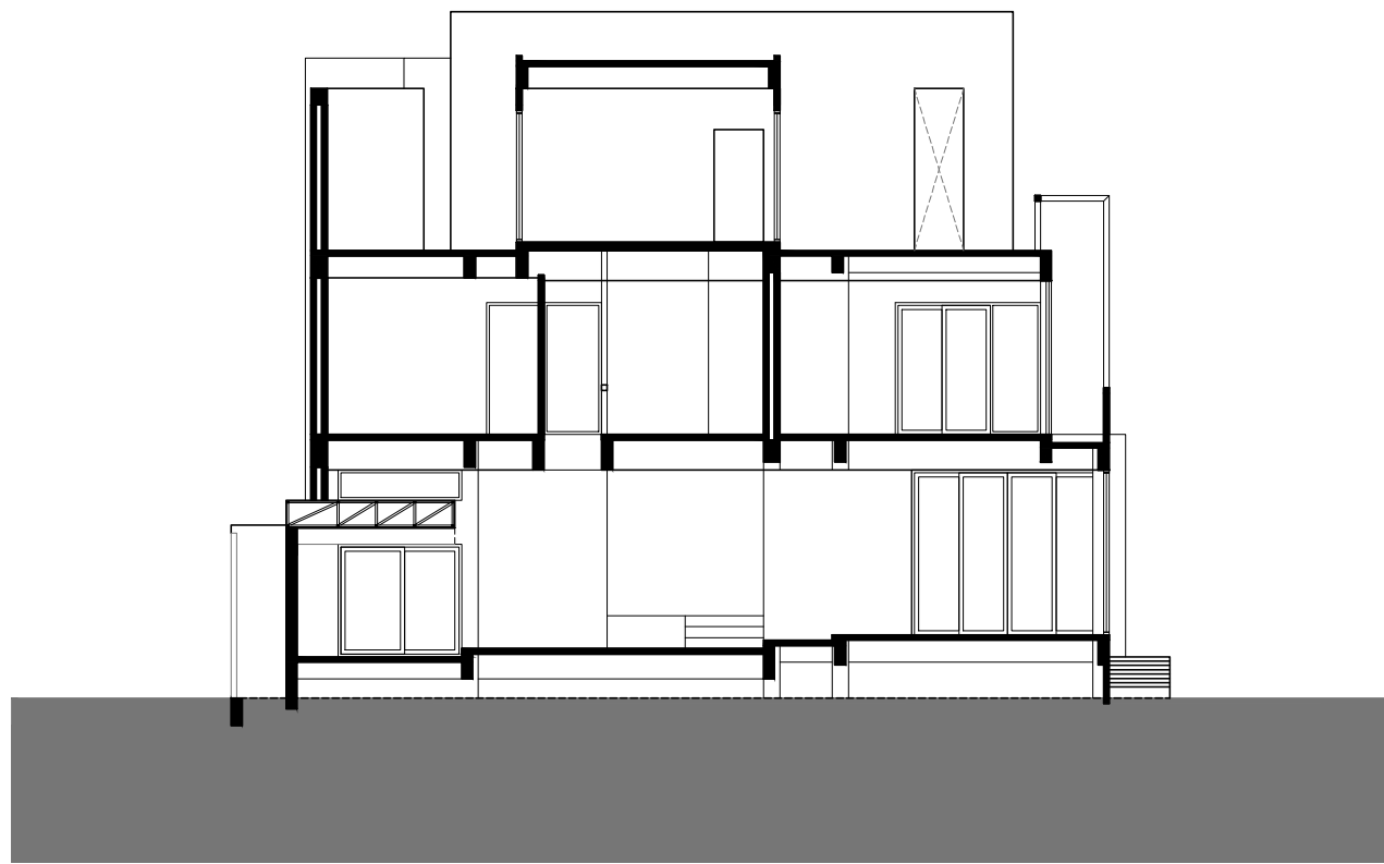
A-A SECTION
