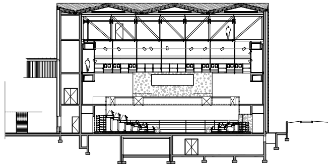
COUPE TRANSVERSALE SUR LA SALLE VERS LA REGIE
