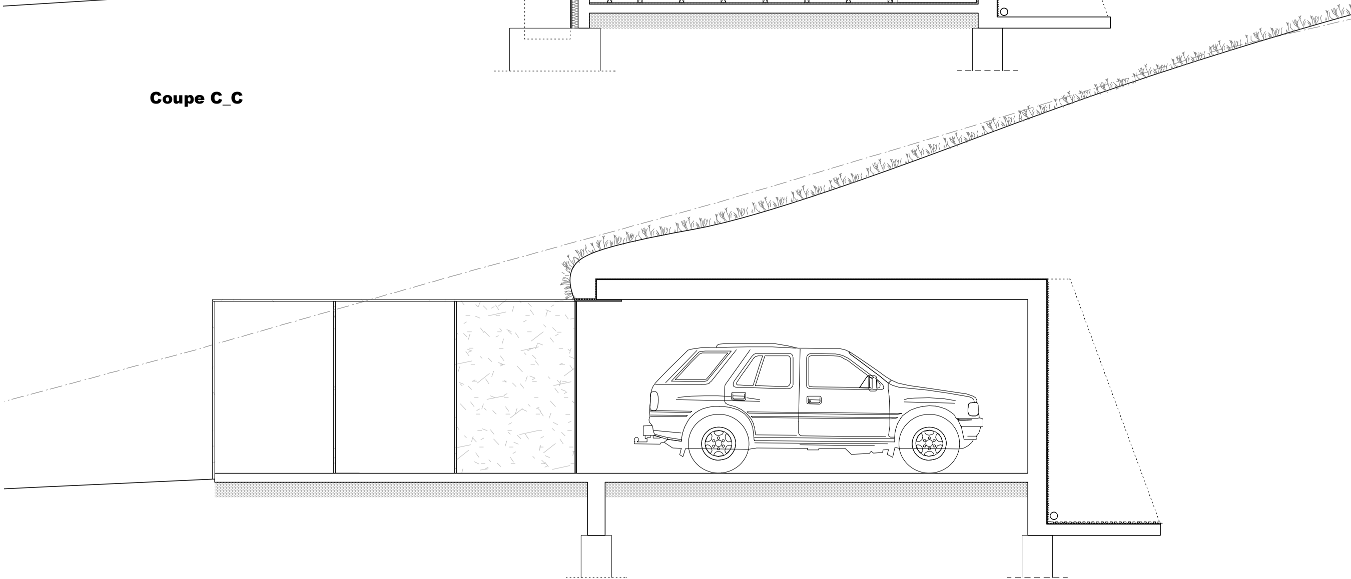
Coupe D_D
