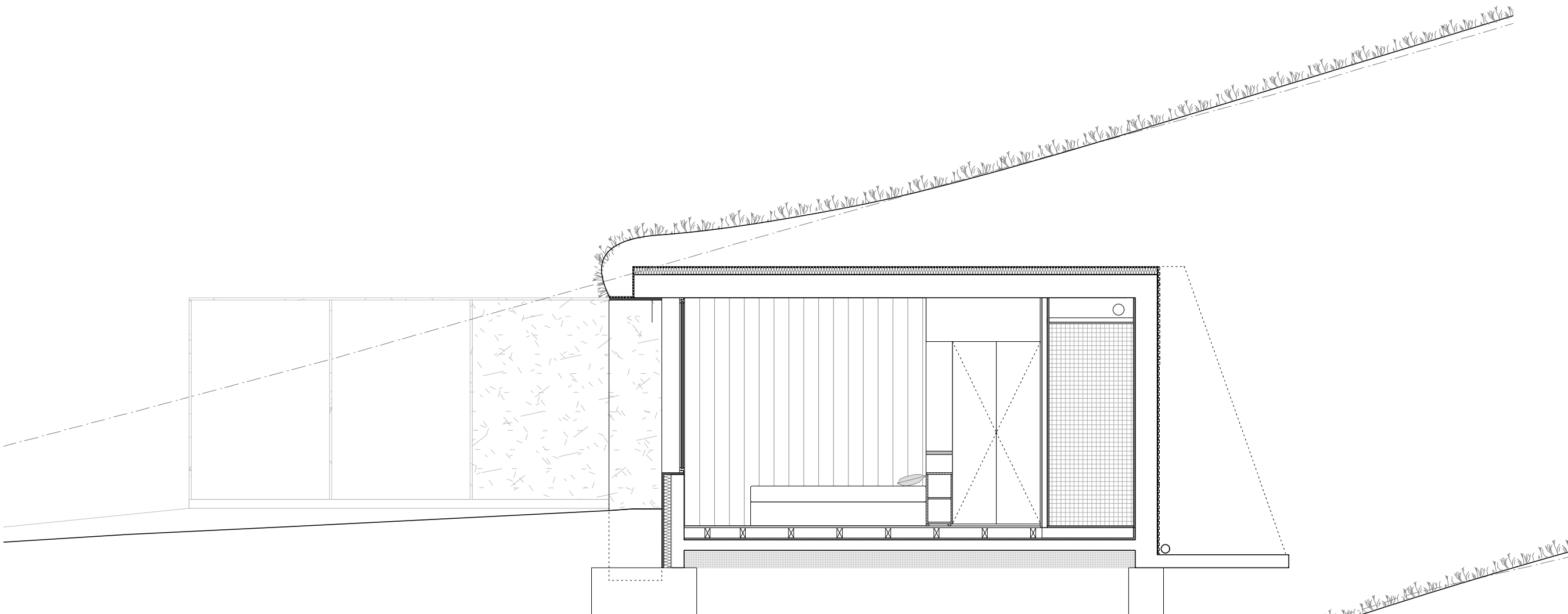
Coupe C_C
