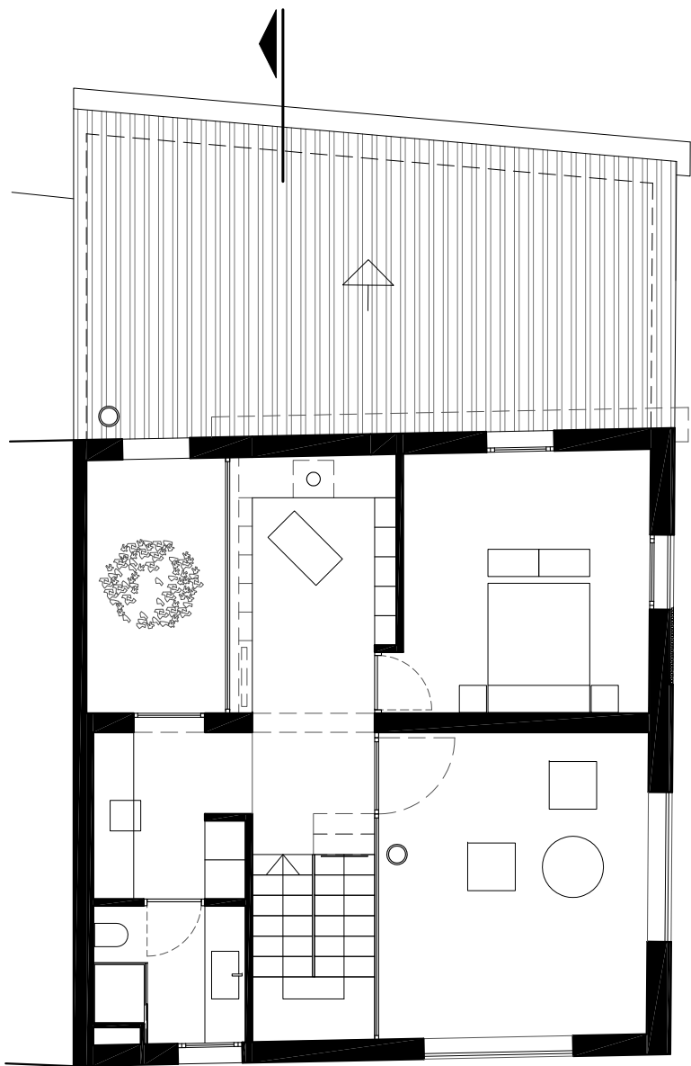
PLANTA SEGONA
