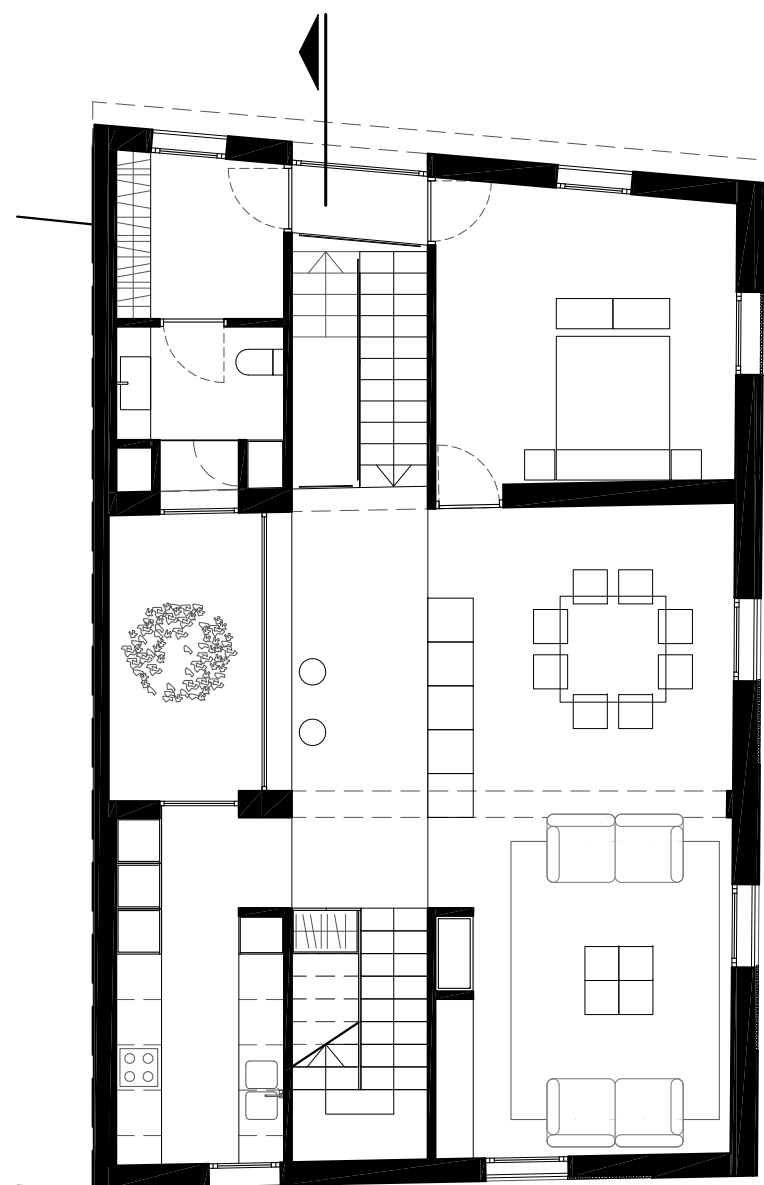
PLANTA PRIMERA
