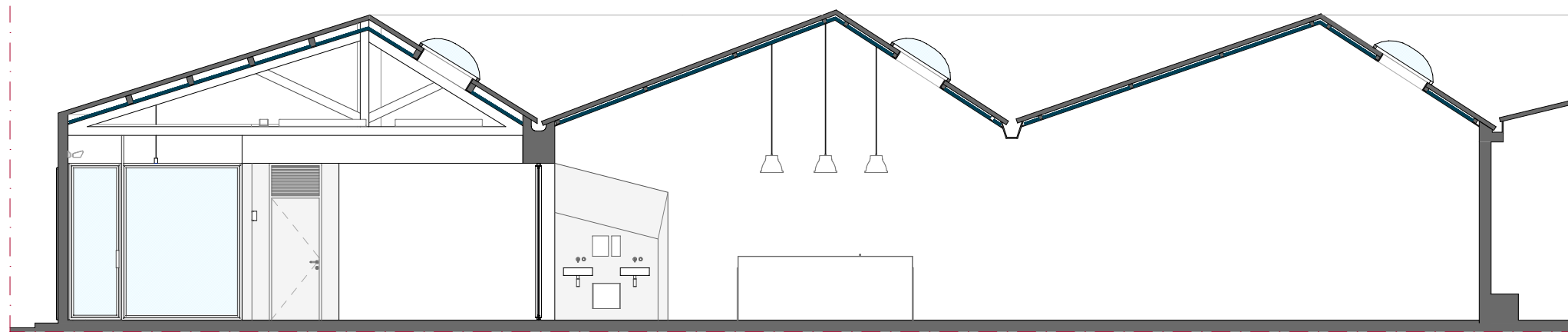
CORTE 09
