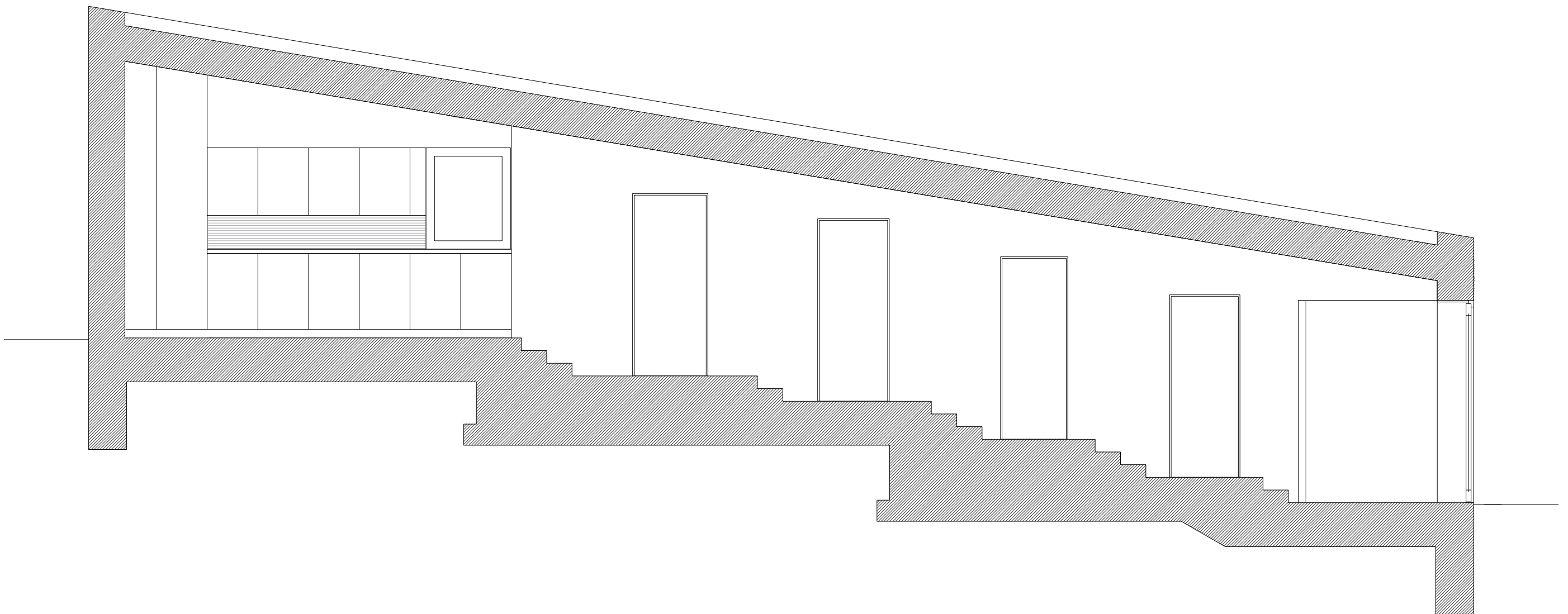
langse snede - schaal 1/50
