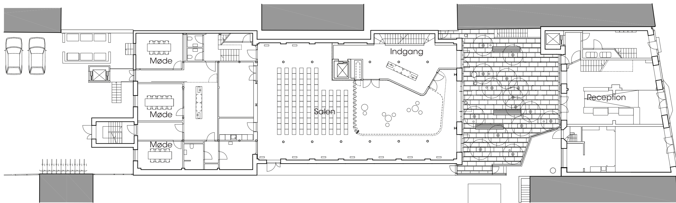
Stueplan 1:200
