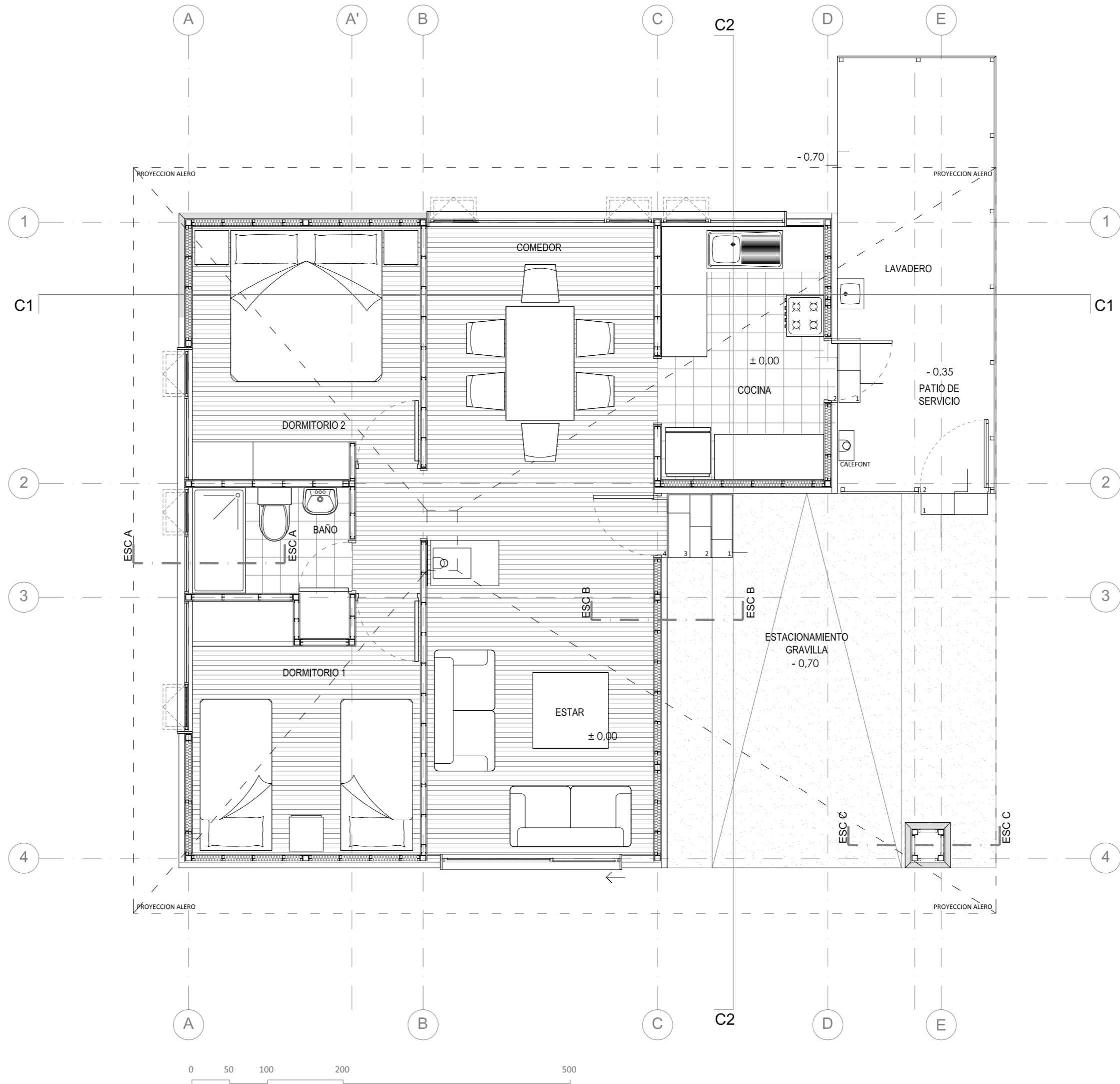
planta 1º nivel
