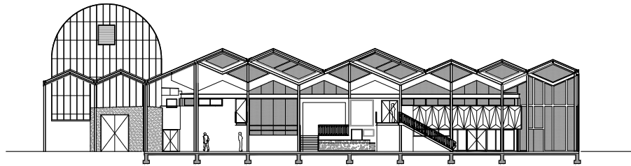
COUPE SUR L'ATRIUM VERS L'EXISTANT
