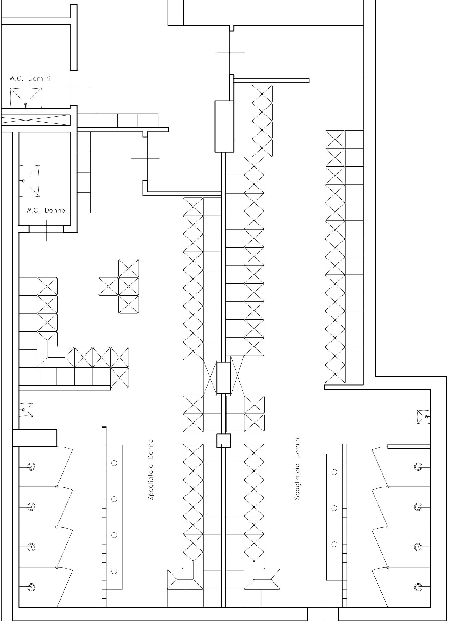
Layout Spogliatoi scala 1:50
