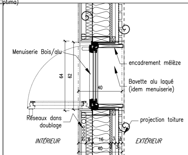
Coupe horizontale sur menuiserie bois
