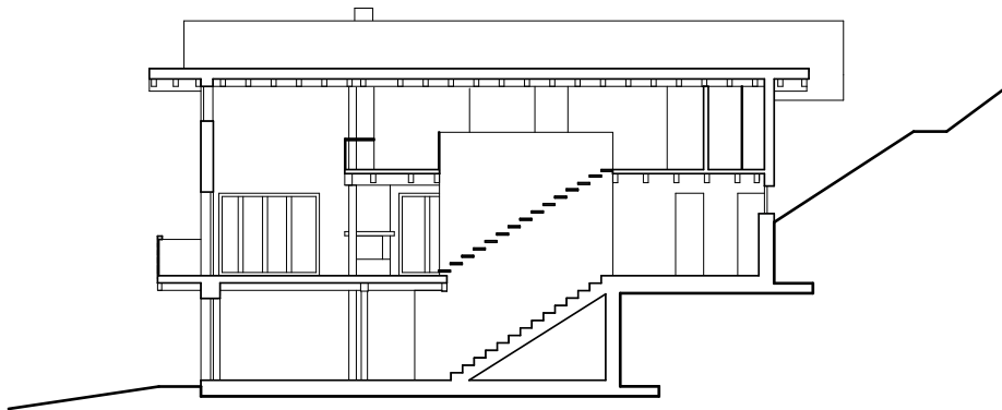
Coupe longitudinal
