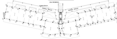
PIANTA PIANO TIPO SCALA 1/50
