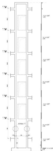
SEZIONE A-A SCALA 1/50
