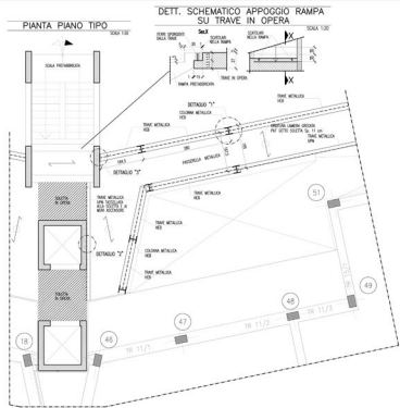
DETTAGLI STRUTTURALI PASSERELLA METALLICA
