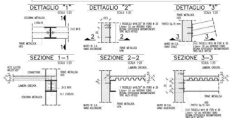
DETTAGLI STRUTTURALI PASSERELLA METALLICA
