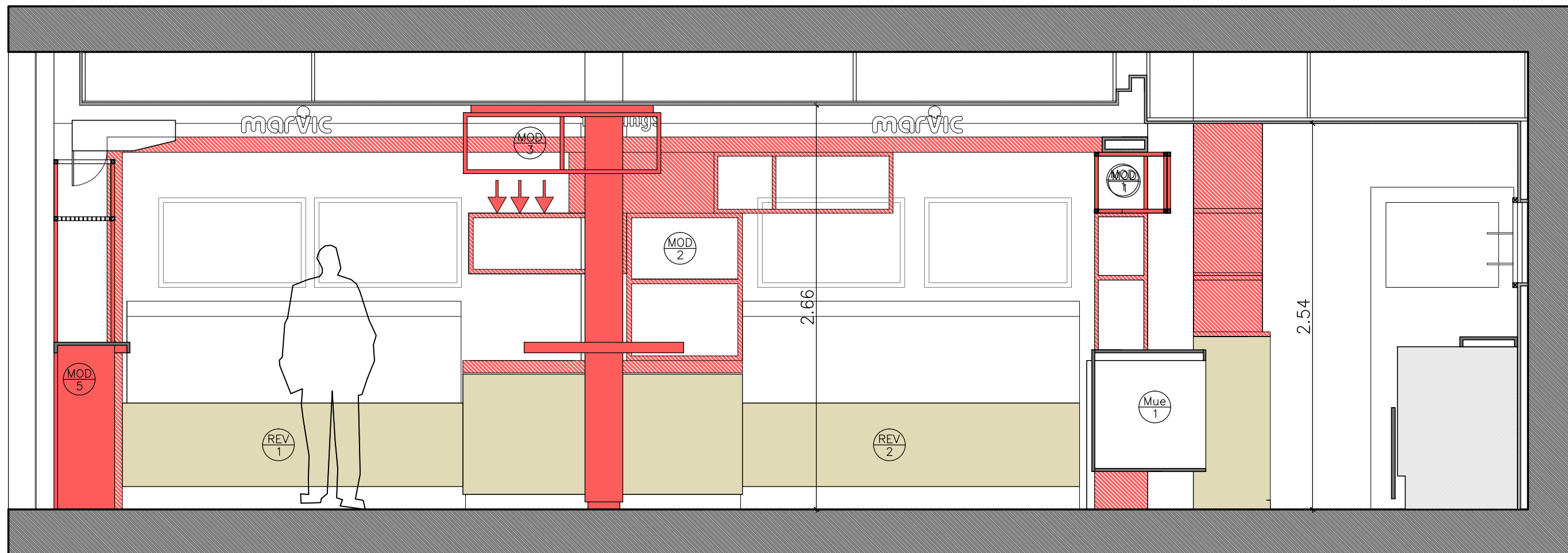
CORTE 1-1
