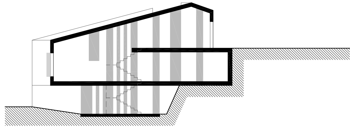
SECCIÓ LONGITUDINAL
