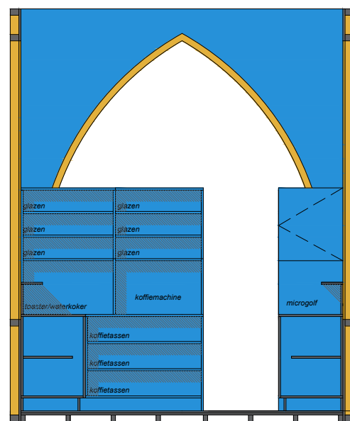
snede A
