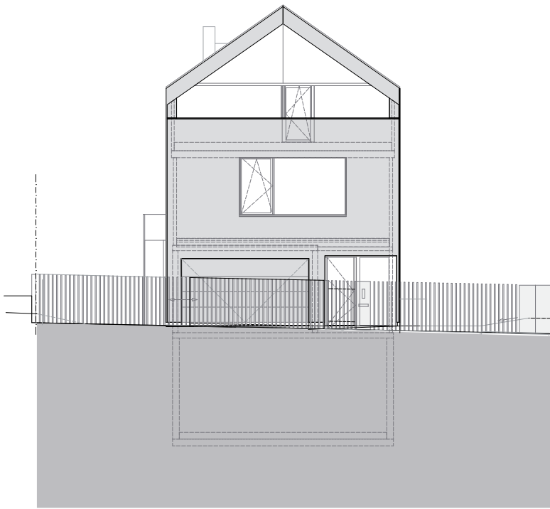
Ansicht Süd 1:200
