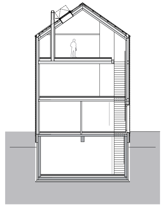
Querschnitt 1:200
