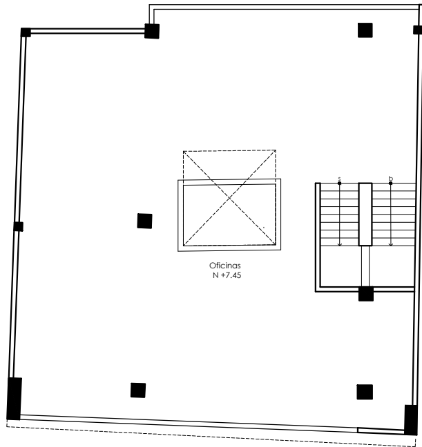
⊙ NIVEL 3
