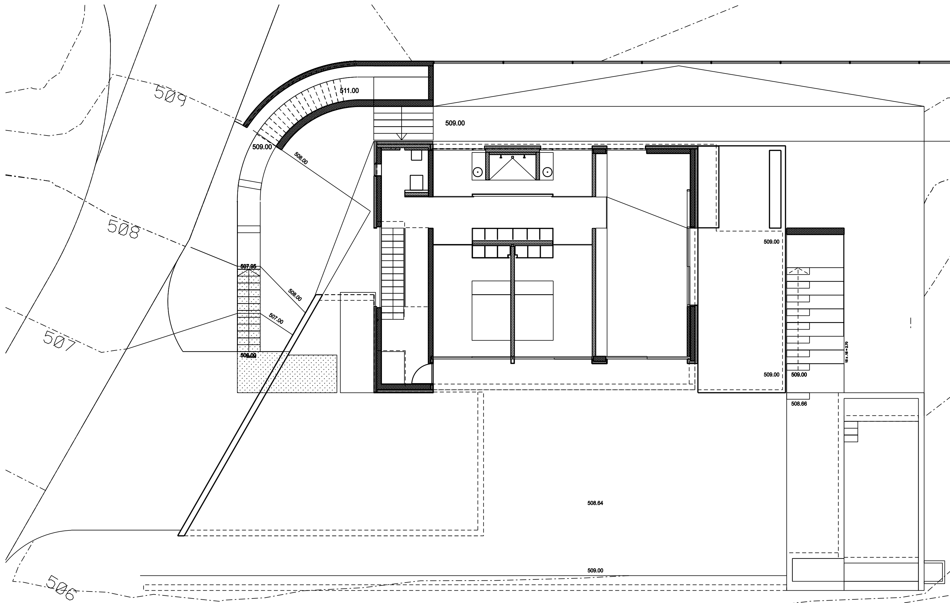
feldbalz house 1:100 groundfloor gus wüstemann ma eth sia coac
