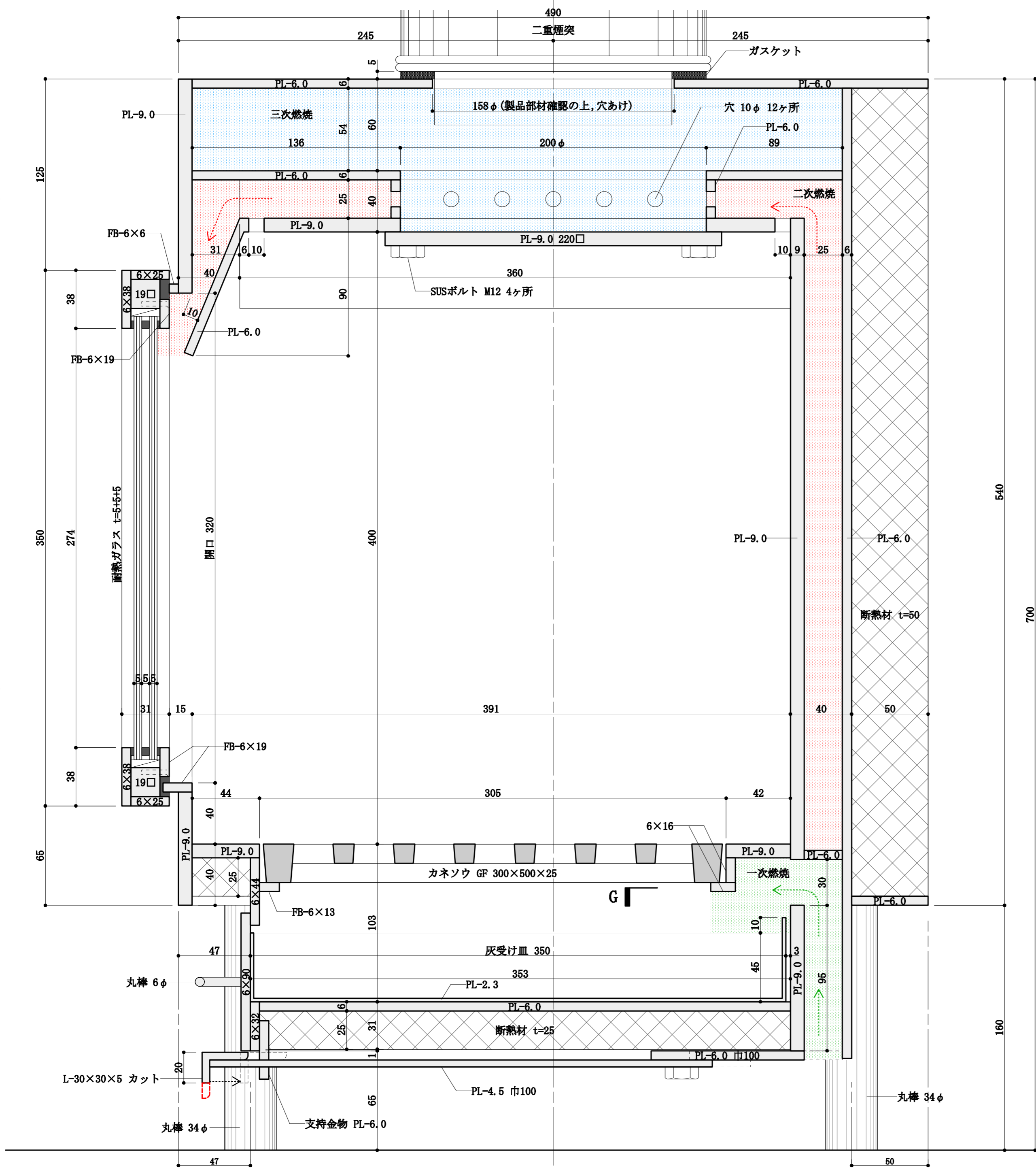
C-C' 断面図 1:2
