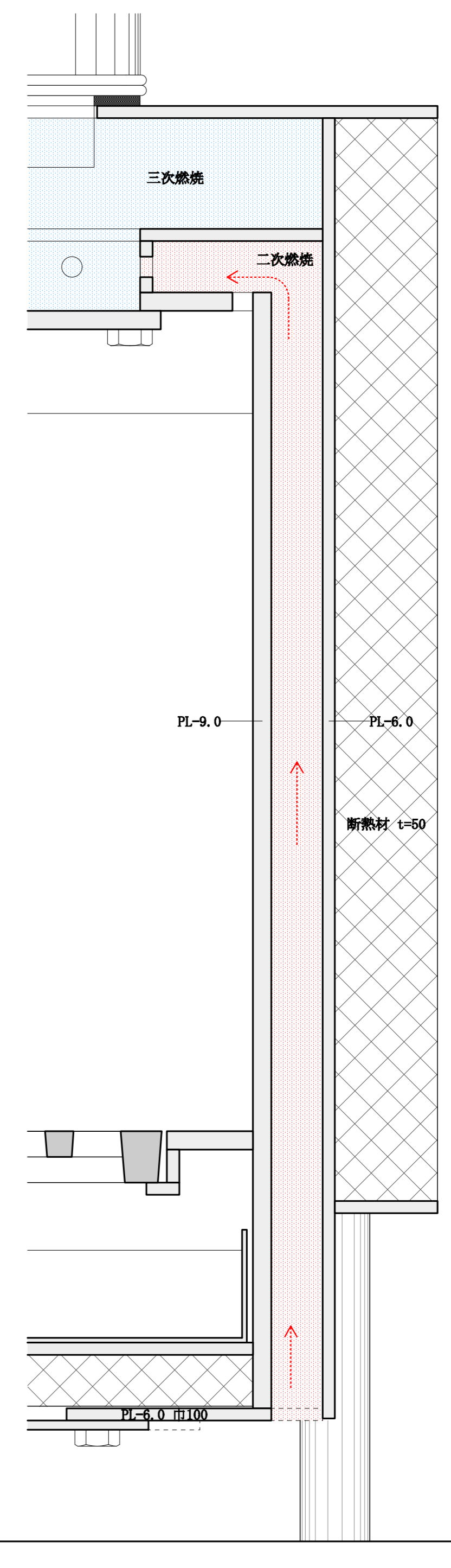
D-D' 断面図 1:2
