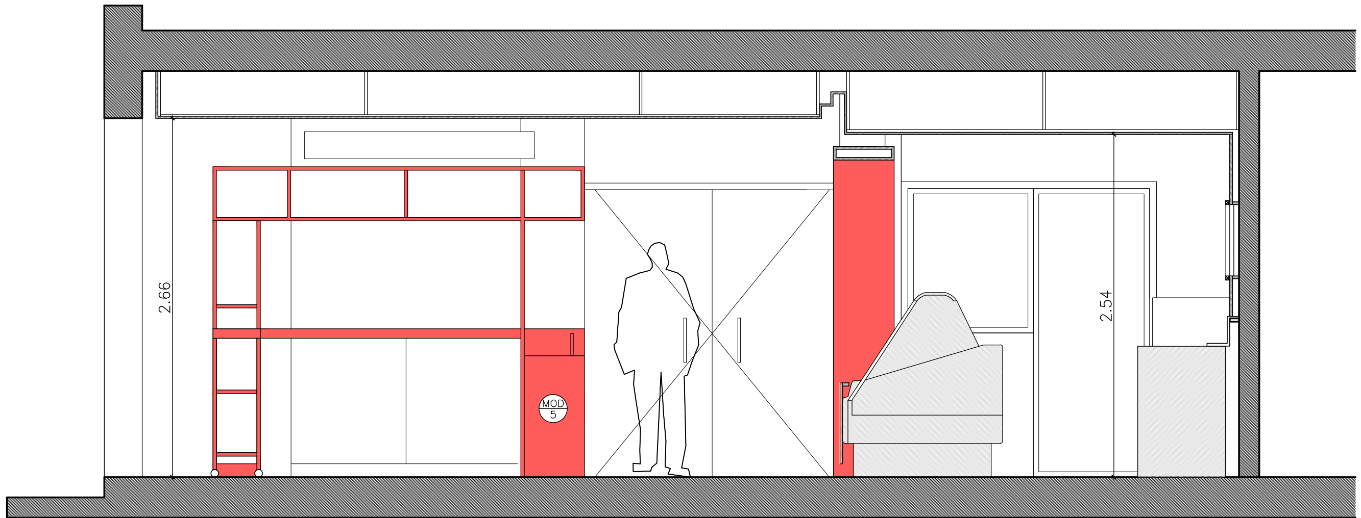
CORTE 7-7
