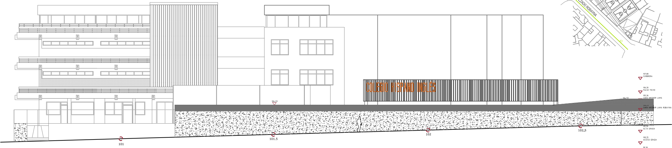
ALZADO A LA RAMBLA
