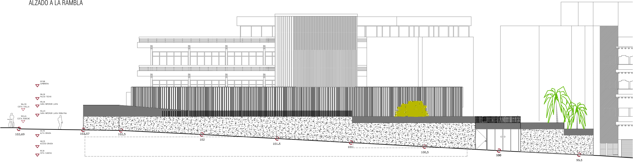
ALZADO A LA RAMBLA
