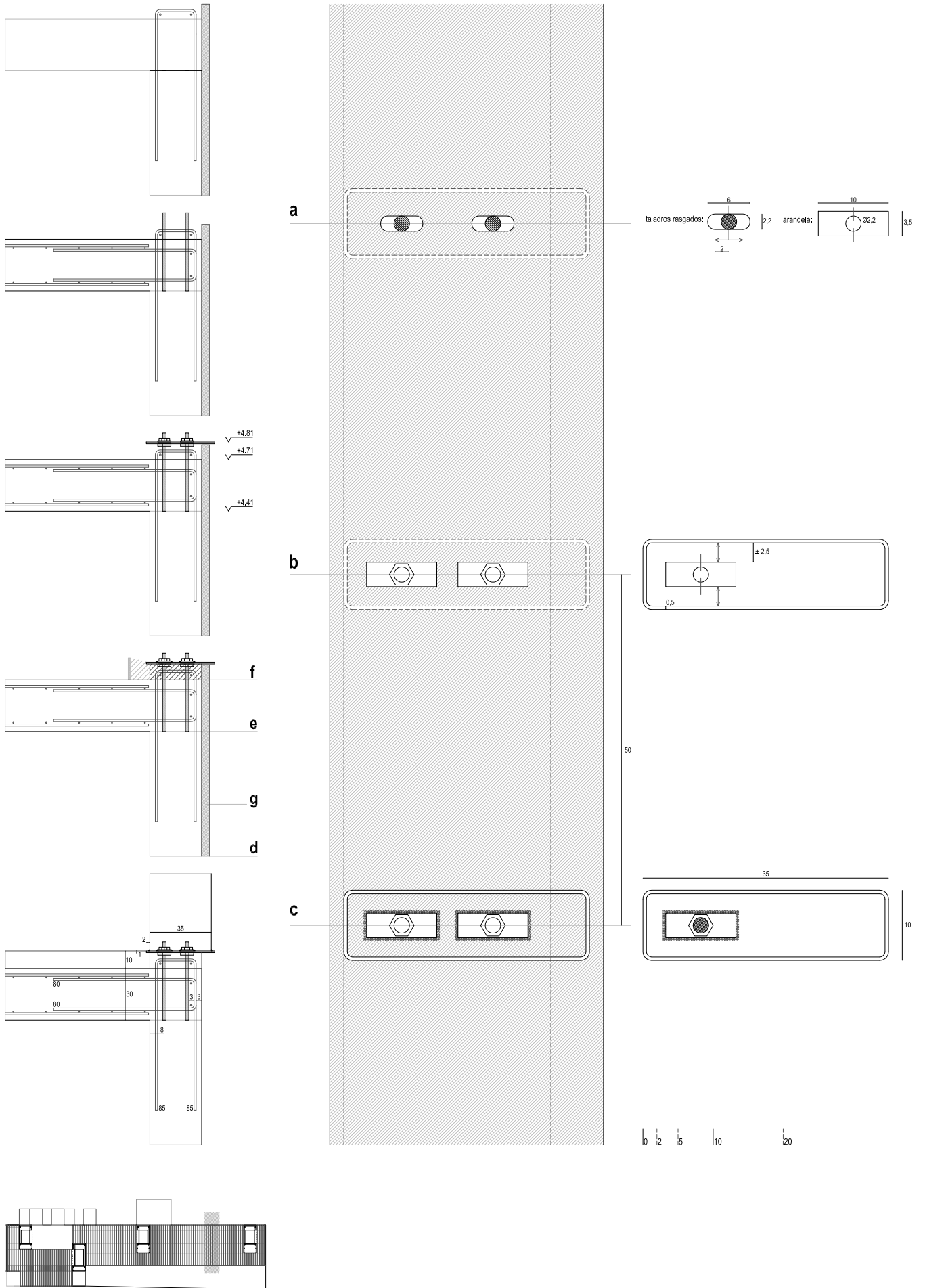
a. REGULACIÓN VERTICAL CON TUERCAS, CON POSIBILIDAD DE MOVER LA CHAPA EN SENTIDO TRANSVERSAL A LA FACHADA \pm 20 MM; AL SER LA CHAPA UN POCO MÁS GRANDE, EL PILAR SE PUEDE MOVER EN ESTA DIRECCIÓN. b. EL ANCHO DEL PILAR PERMITE MOVERLO \pm 25 MM. c. LA ANCHURA DE LA CHAPA AUMENTA LA TOLERANCIA Y PERMITE SOLDAR MEJOR EL SOPORTE. LA ARANDELA SE SUELDA A LA CHAPA TRAS LA REGULACIÓN. d. HORMIGONADO 1°. e. HORMIGONADO 2° (CON CHAPA DEFINITIVA). f. HORMIGÓN HA-25 CON SUPER FLUIDIFICANTE (A/C MUY BAJA). g. EL ENCOFRADO EXTERIOR SE APROVECHA PARA EL TACÓN DE 10 CM.
