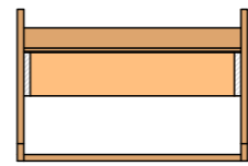
Prospetto B-B
