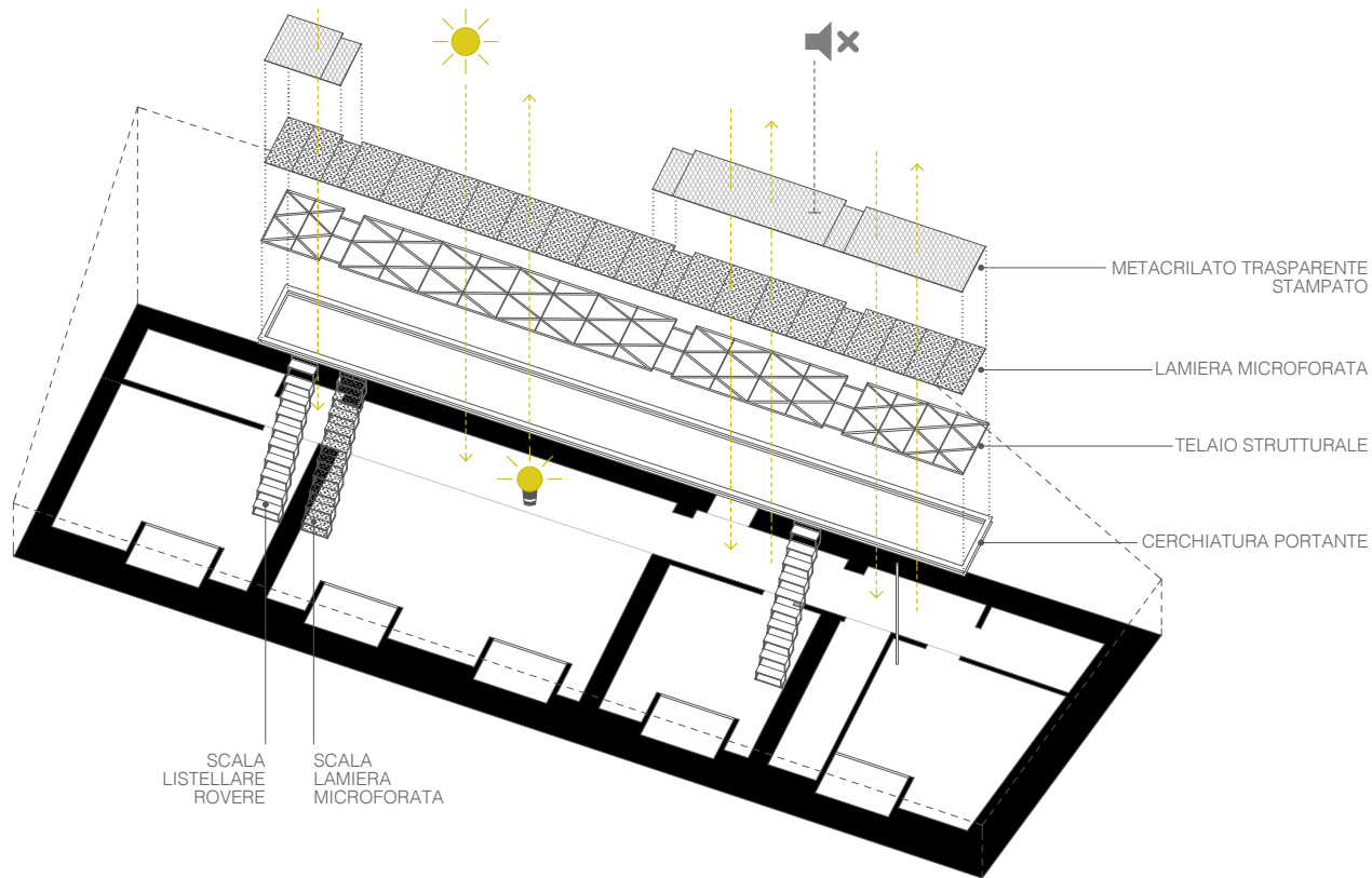
SOPPALCO E COLLEGAMENTI VERTICALI_ESPLOSO ASSONOMETRICO
