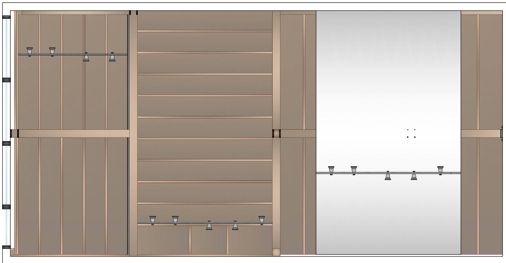
ПЛАФОН 2 M= 1:50
