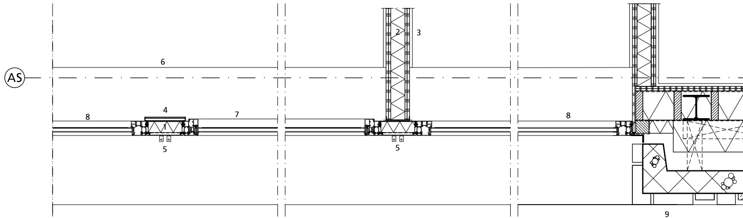
2e verdieping
