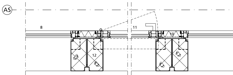
begane grond
