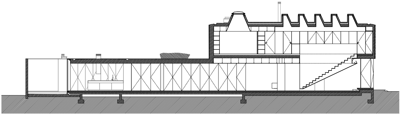
SECTION DD
